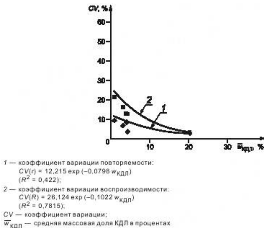
Рисунок А.4 — Коэффициенты вариации повторяемости CV(r) и воспроизводимости CV(R) для определения КДЛ
