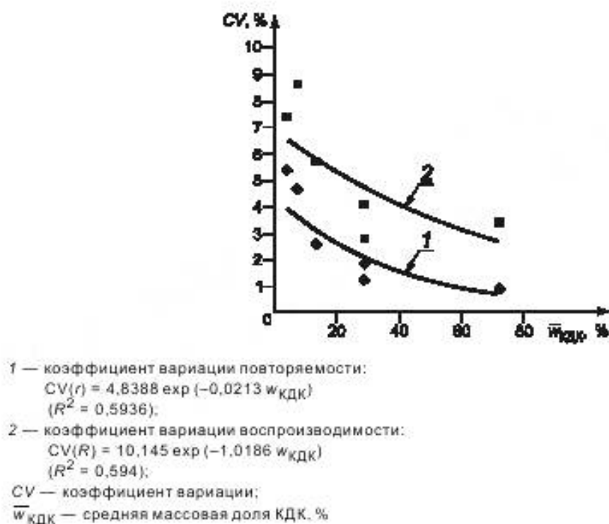
Рисунок А.3 — Коэффициенты вариации повторяемости CV(r) и воспроизводимости CV(R) для определения КДК
