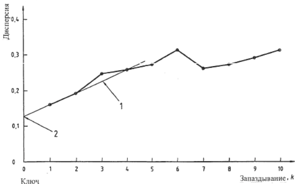
Рисунок 3 Вариограмма для данных из таблицы А.2
