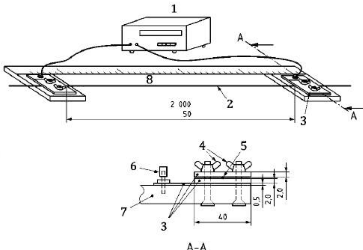
1 — измеритель сопротивления; 2 — образец для испытаний; 3 — электрод (медный); 4 — скрепляющая гайка; 5 — образец для испытаний; 6 — вывод (контакт); 7 — изолирующая пластина; 8 — измеритель длины
