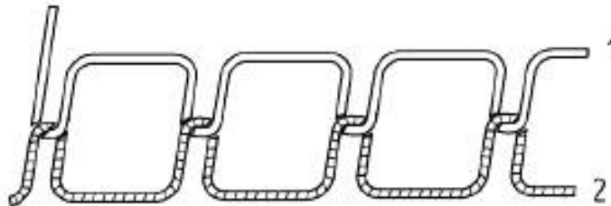
1 – игольная нитка, 2 – шпулечная нитка
