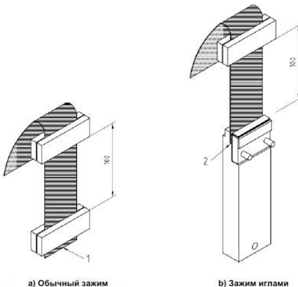
Рисунок 2 – Положение образца для испытаний
