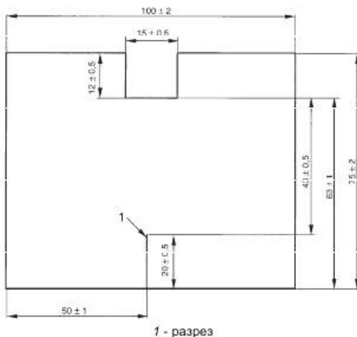
Рисунок 1— Размеры испытуемого образца
