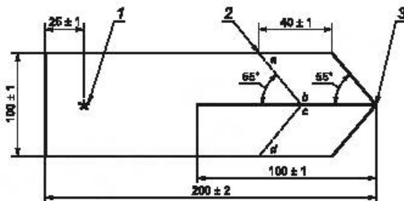
Рисунок 1 — Испытуемый образец в форме крыльев
