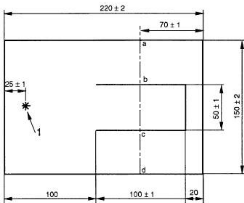
Рисунок 2 – Испытуемый образец в форме языка
