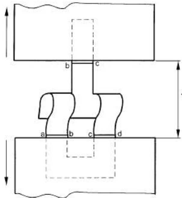
Рисунок 3 — Расположение зажимов
