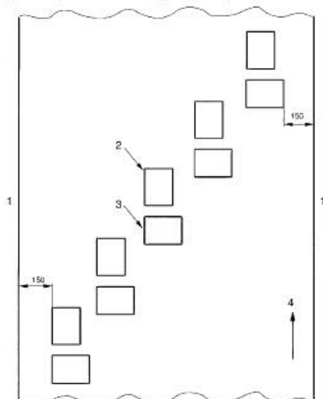
1 – край; 2 – пробы для раздиранья «поперек основы»; 3 – пробы для раздиранья «поперек утка»; 4 – основа
