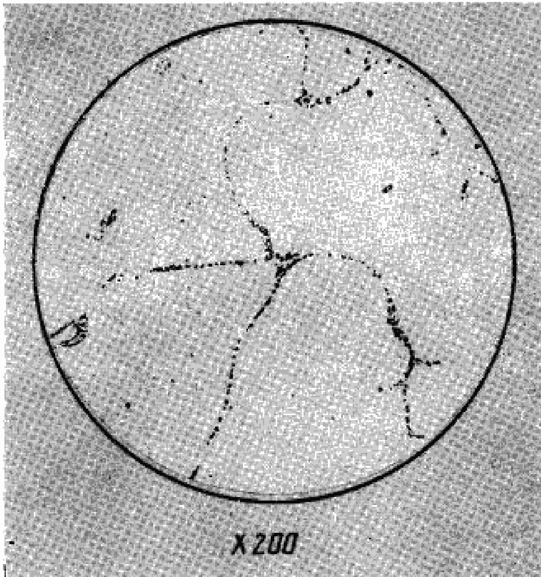
Черт. 7. Материал — литейная медь, массовая доля кислорода — 0,015%, освещение — рассеянный свет
