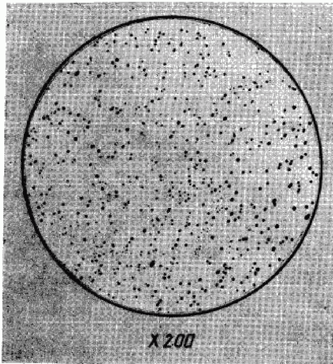
Черт. 4. Материал — деформированная медь, массовая доля кислорода — 0,00 %, освещение — рассеянный свет
