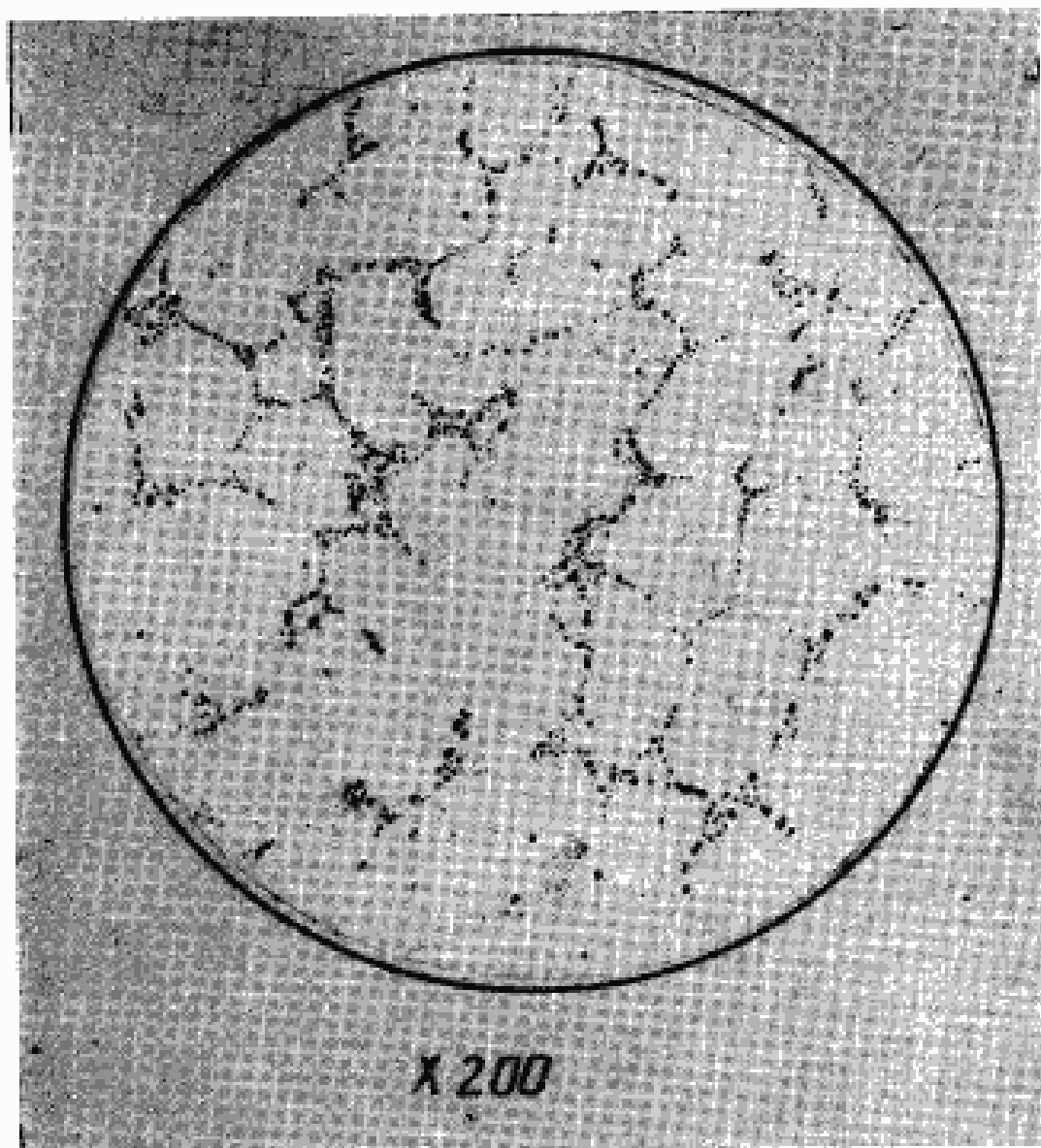
Черт. 10. Материал — литая медь, массовая доля кислорода — 0,05%, освещение — рассеянный свет
