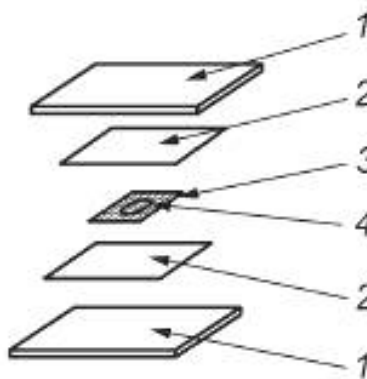
1 — плита пресса; 2 — полиэфирная пленка; 3 — хромникелевая сетка; 4 — образец
