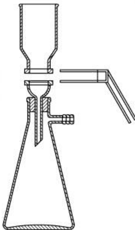
Рисунок 2 — Вакуумная фильтровальная система
