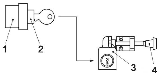
а) Под напряжением с отказом в доступе
