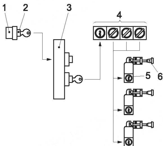
а) Временная задержка, обменный ящик и многократный вход — включено при отказе в доступе
