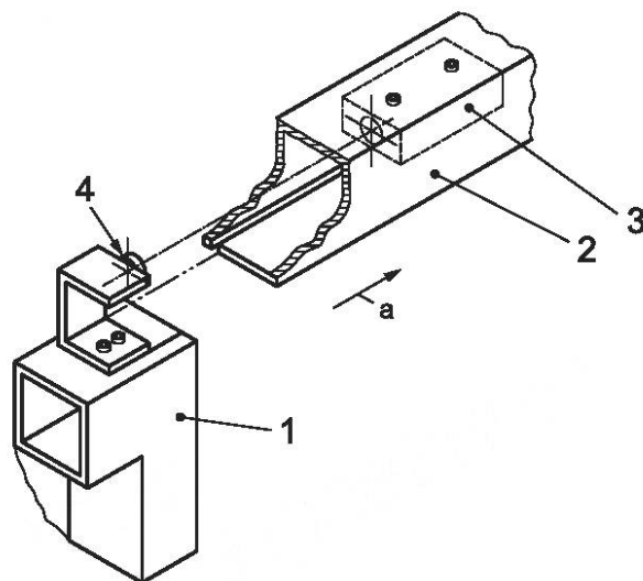
б) Низкоуровневое кодированное блокировочное устройство Типа 3 или 4
