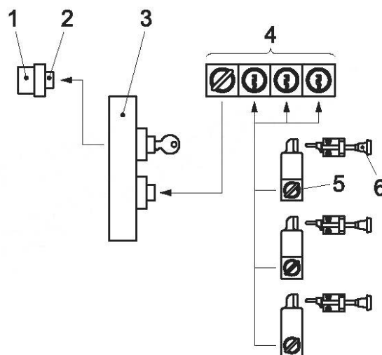
б) Задержка времени, обменный бокс и многократный вход — обесточены с включенным доступом
