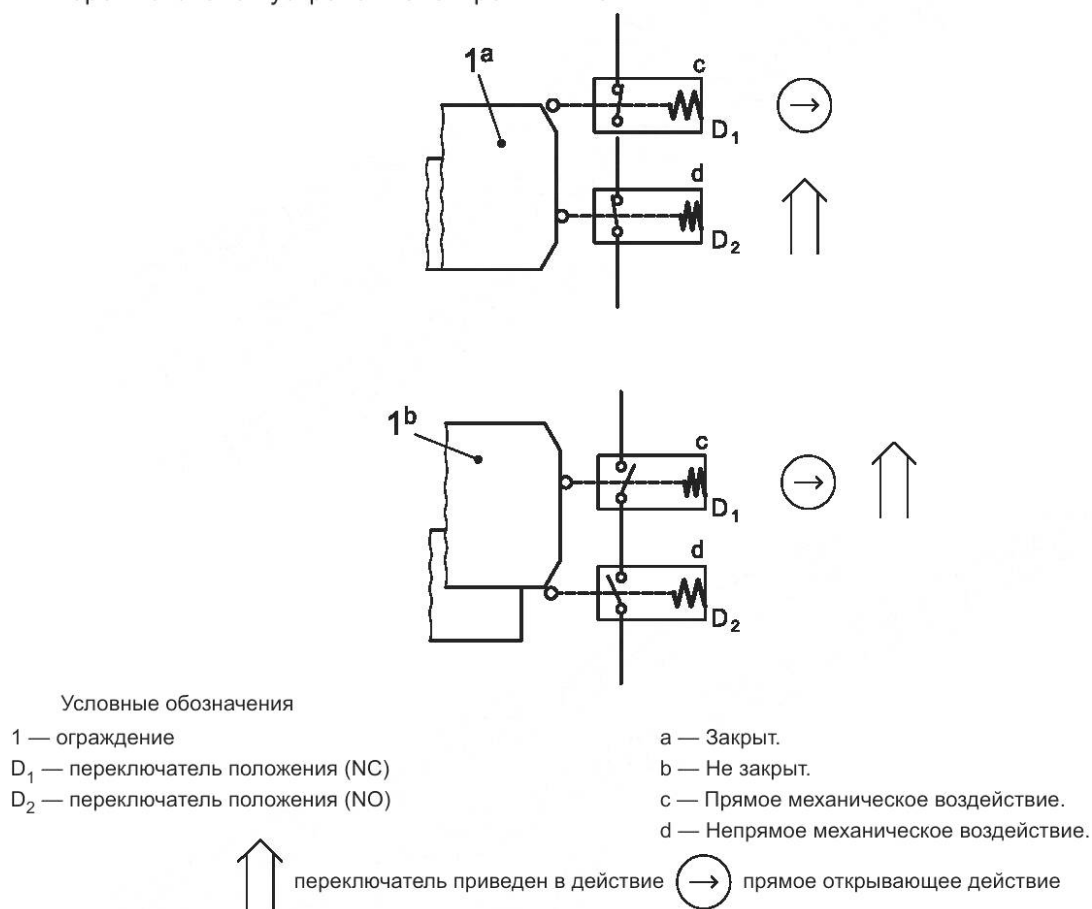
Рисунок 12 — Предотвращение выхода из строя по общей причине двух переключателей положения с механическим приводом за счет использования соответствующего прямого и непрямого механического воздействия
