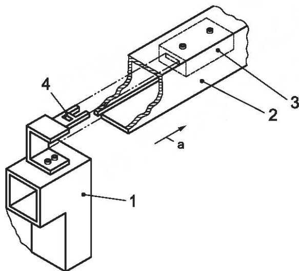
а) Блокировочное устройство Типа 2
