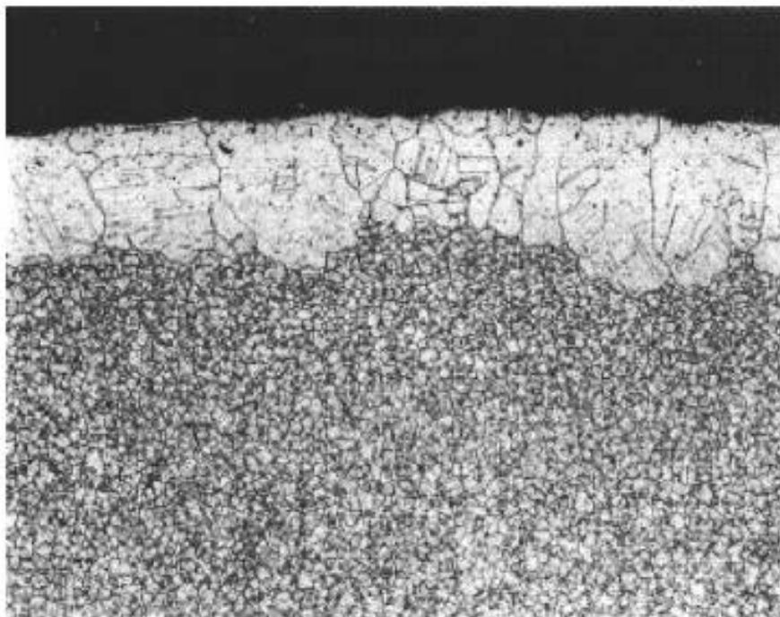
Рисунок 4 – CS размер зерна
