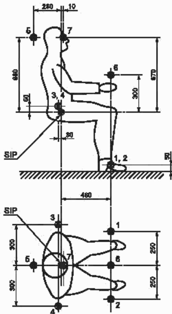
Рисунок 2 — Расположение точек измерения
