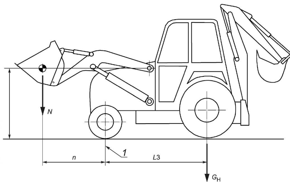
Рисунок 2 — Экскаватор-погрузчик
