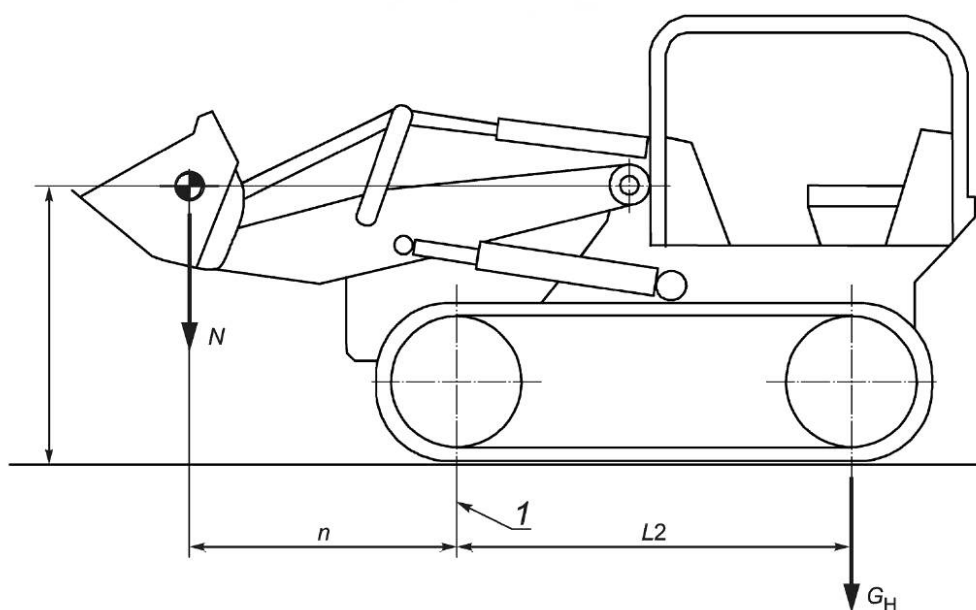
1 — линия опрокидывания
