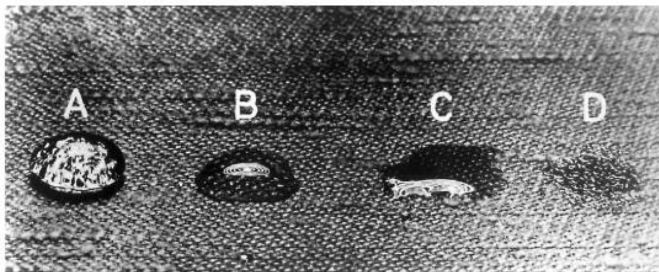
А — маслoneпроницаемость: четкая, округлая капля; В — неполная маслoneпроницаемость: капля, окруженная частичным потемнением; С — проникаемость масла: очевидное растекание и/или полное смачивание; D — проникаемость масла: полное смачивание
