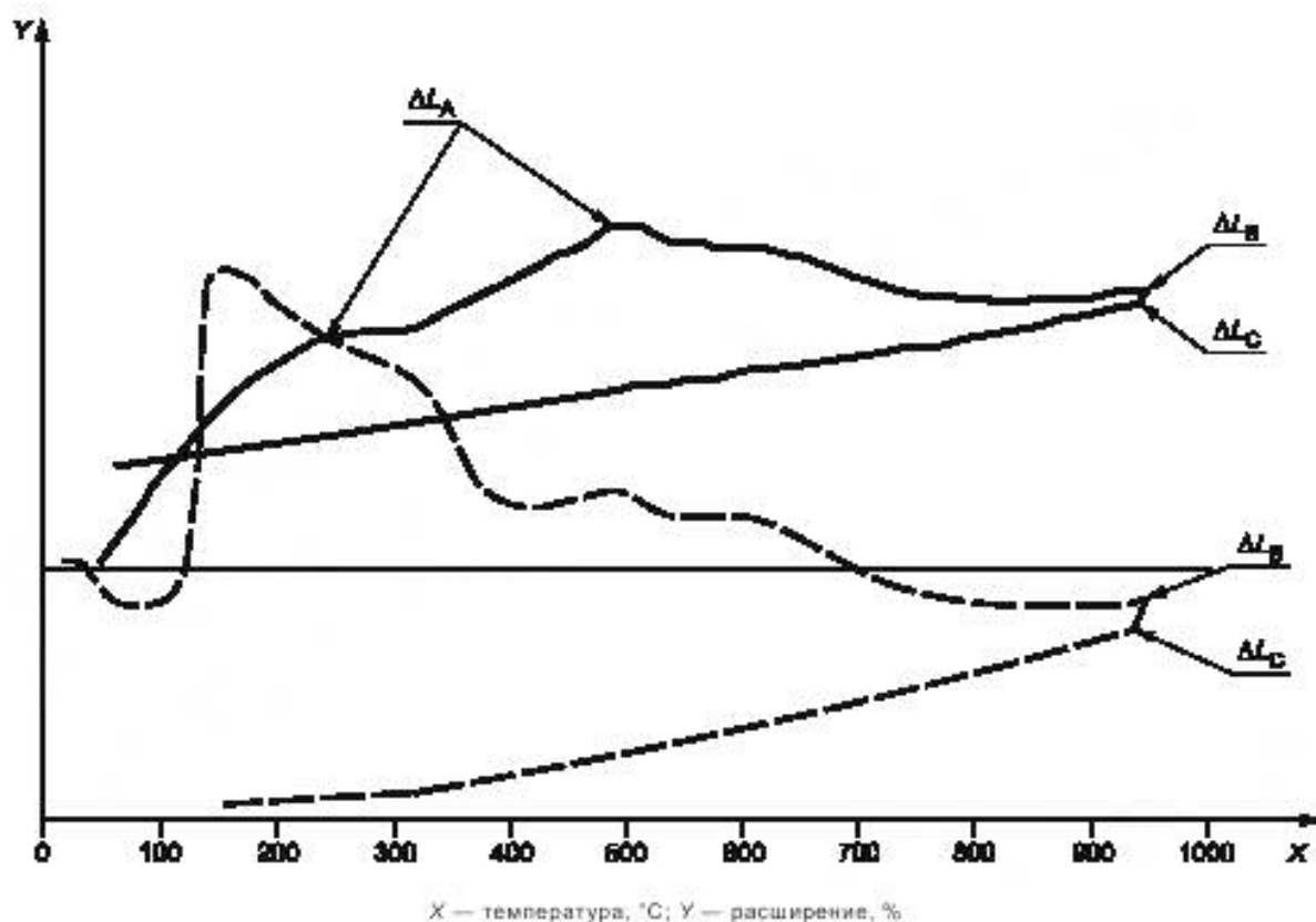
Рисунок 2 — Пример записи зависимости изменения длины от температуры
