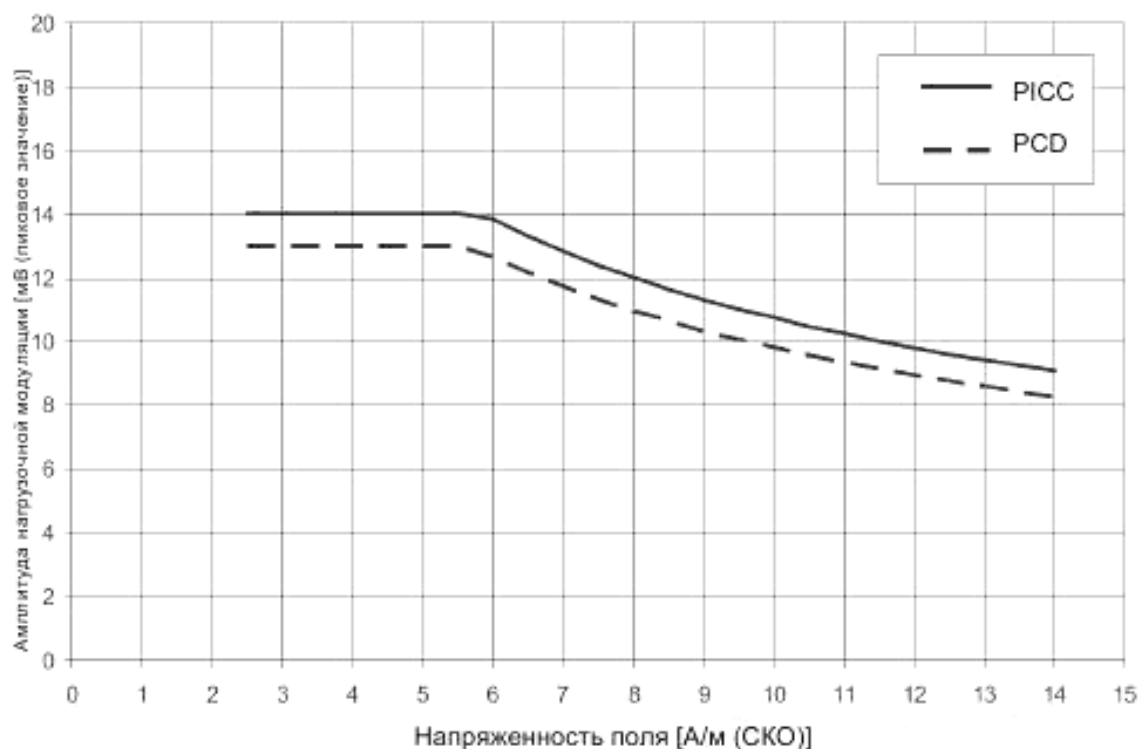
Рисунок 14 – Предельные значения амплитуды нагрузочной модуляции для «Класс 5»
