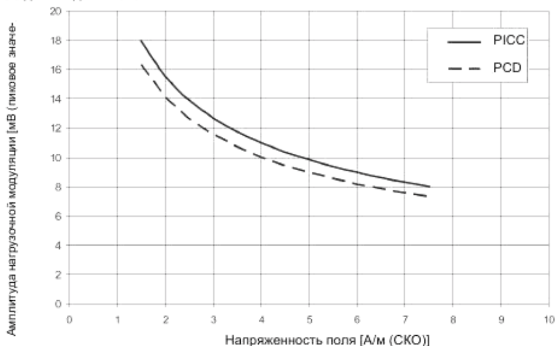
Рисунок 11 – Предельные значения амплитуды нагрузочной модуляции для «Класс 1»
