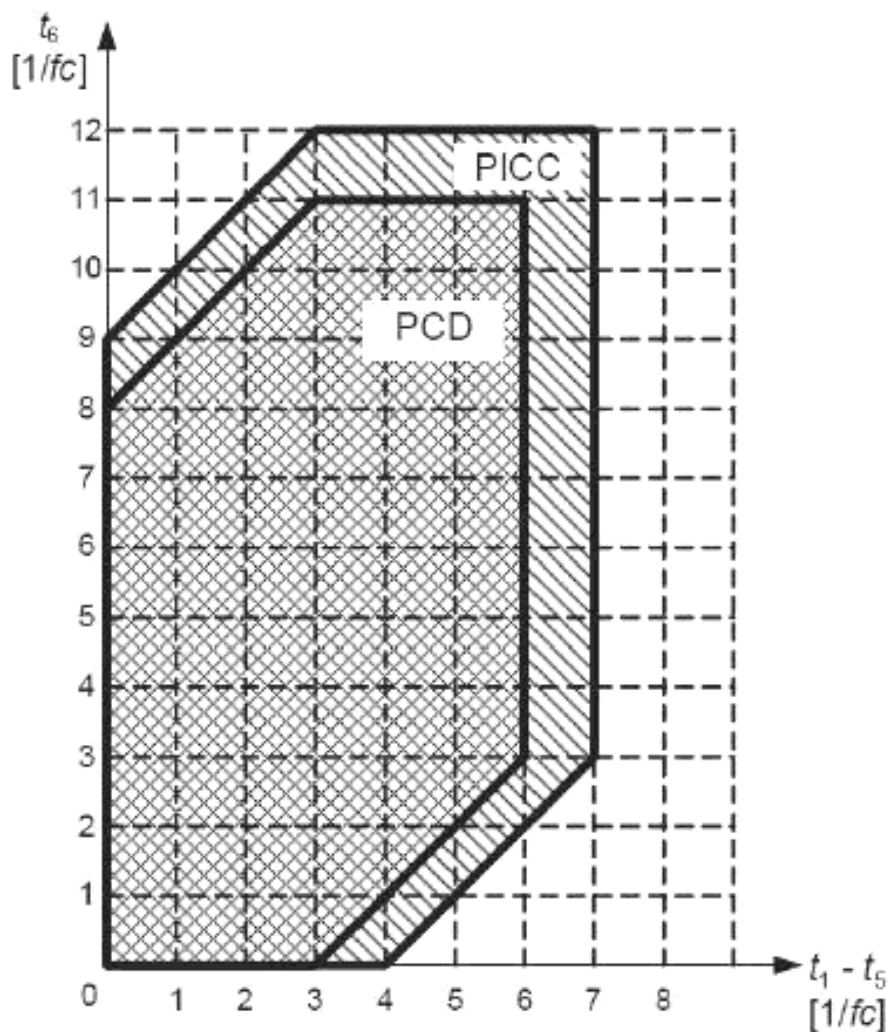
Рисунок 7 – Временные параметры PauseA при скорости передачи fc/64
