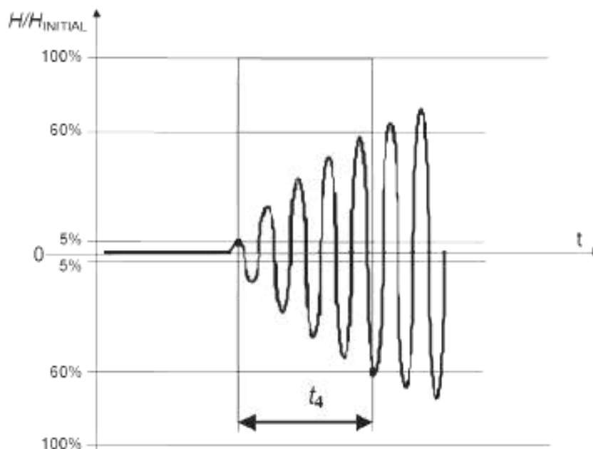
Рисунок 5 – Конец PauseA при скорости передачи fc/128
