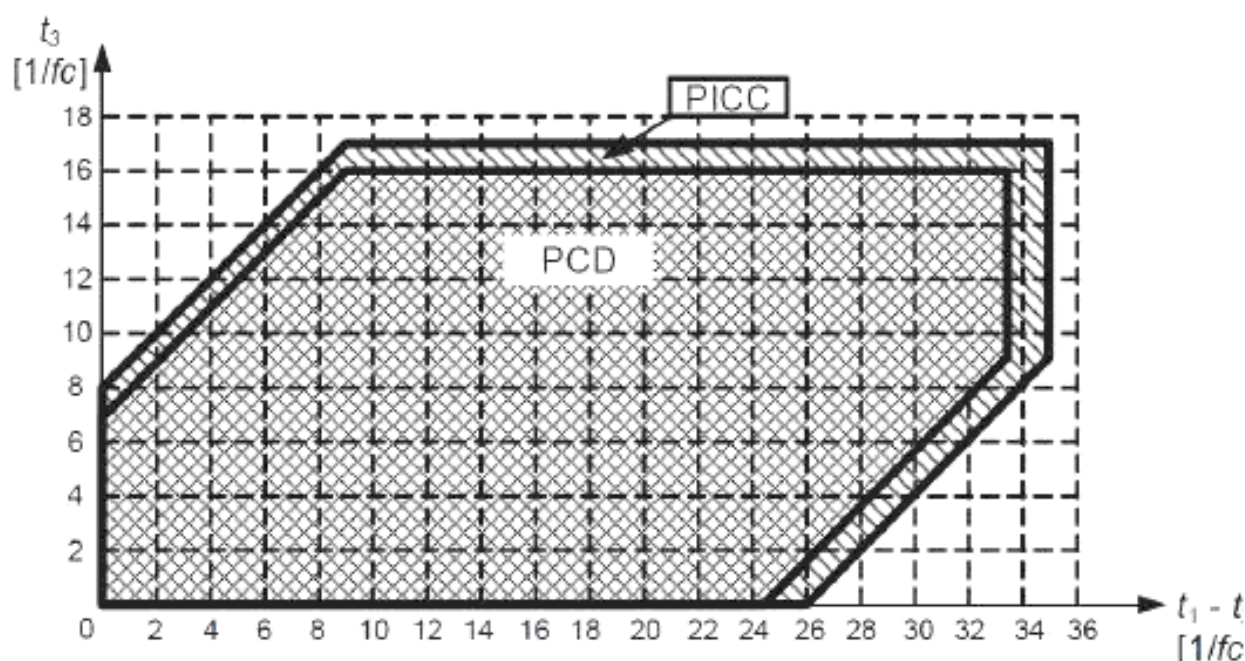
Рисунок 4 – Временные параметры PauseA при скорости передачи fc/128
