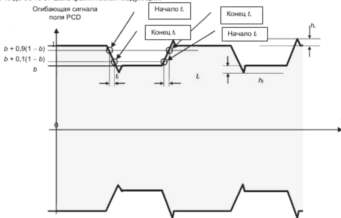
Рисунок 16 – Колебательный сигнал типа В
