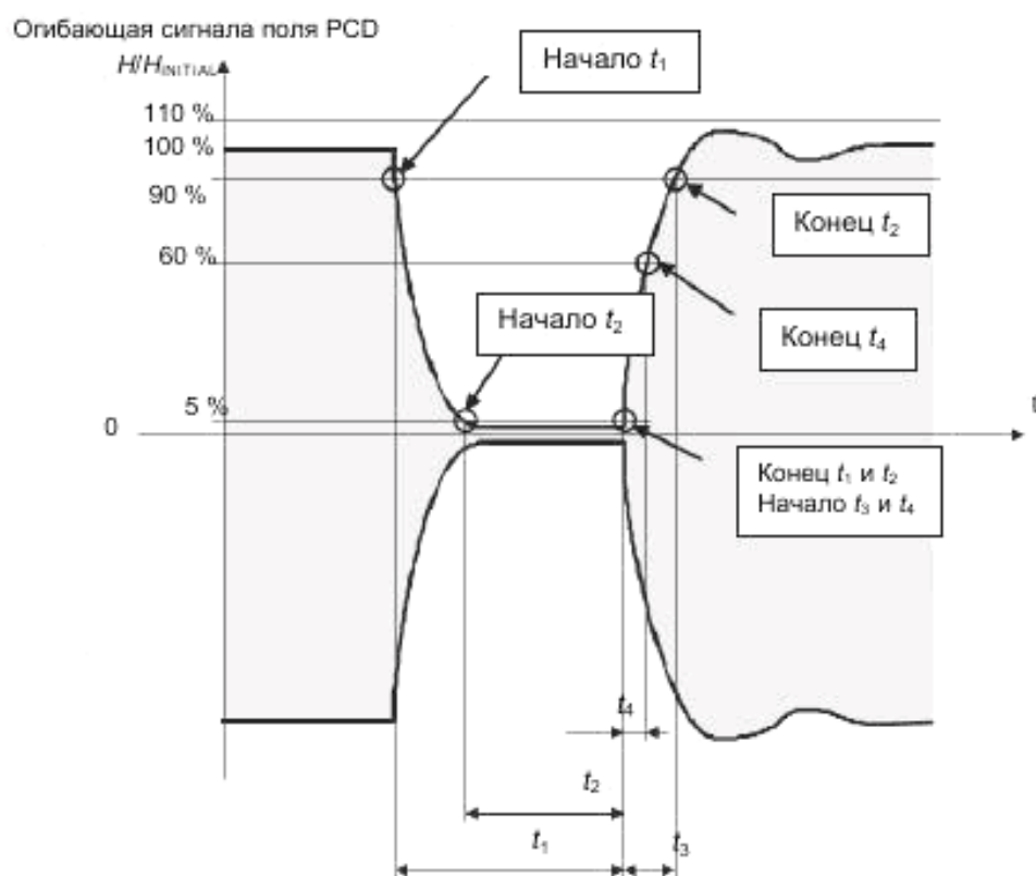
Рисунок 3 – PauseA при скорости передачи fc/128
