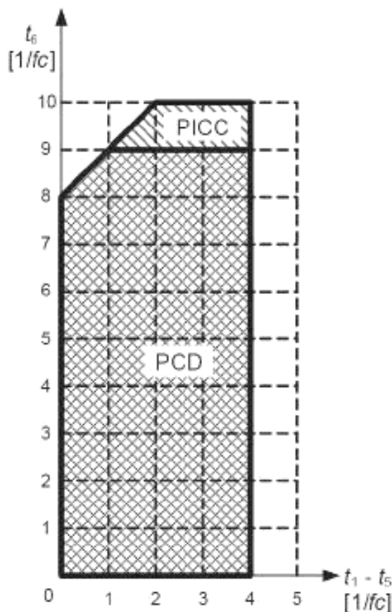
Рисунок 8 – Временные параметры PauseA при скорости передачи fc/32
