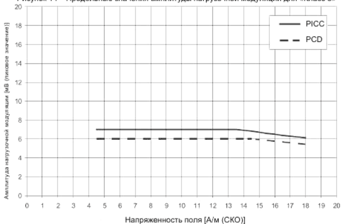
Рисунок 14 – Предельные значения амплитуды нагрузочной модуляции для «Класс 5»
