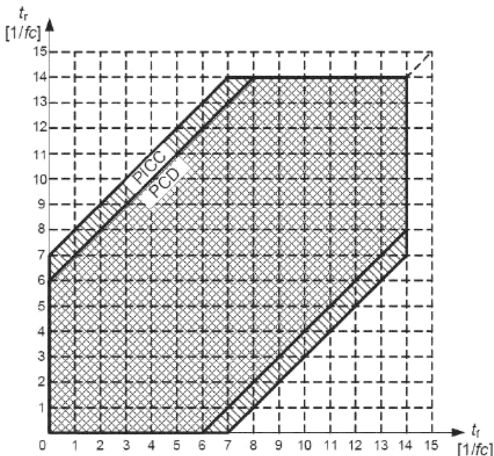
Рисунок 19— Параметры синхронизации модулированного колебательного сигнала типа В
