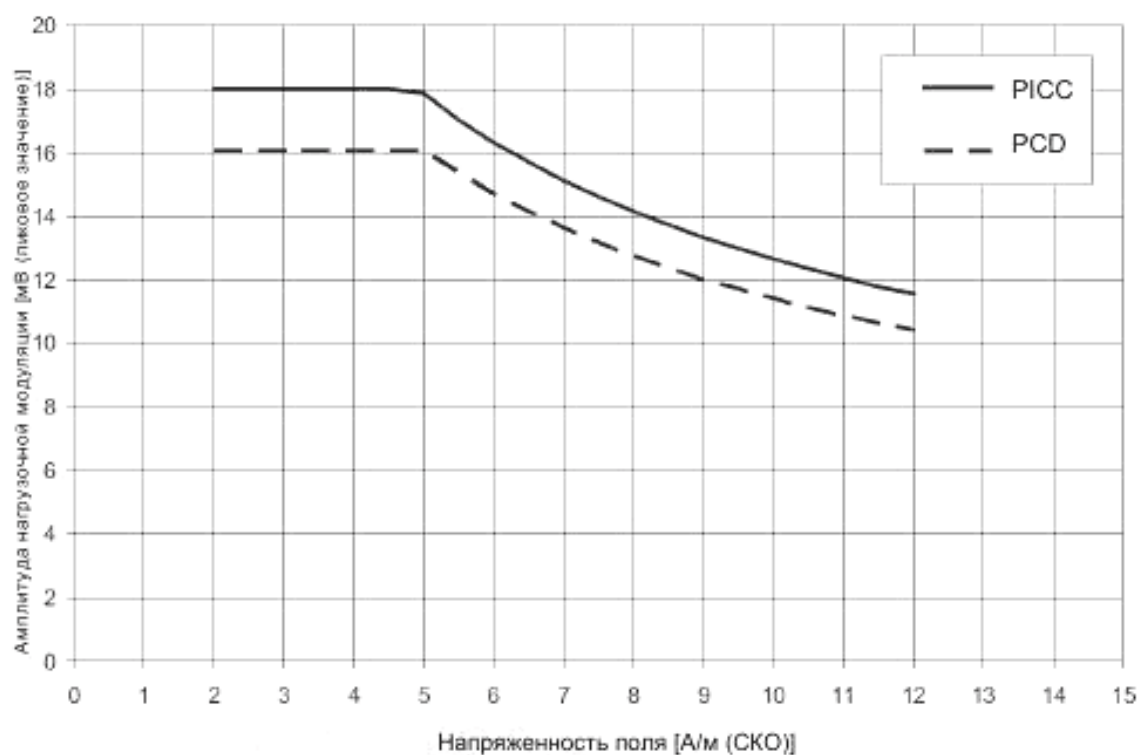
Рисунок 13 – Предельные значения амплитуды нагрузочной модуляции для «Класс 4»
