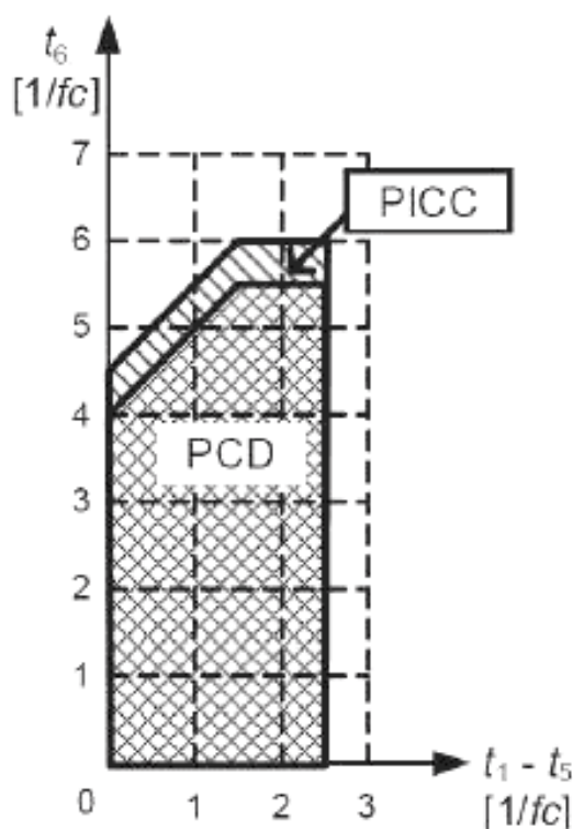
Рисунок 9 – Временные параметры PauseA при скорости передачи fc/16
