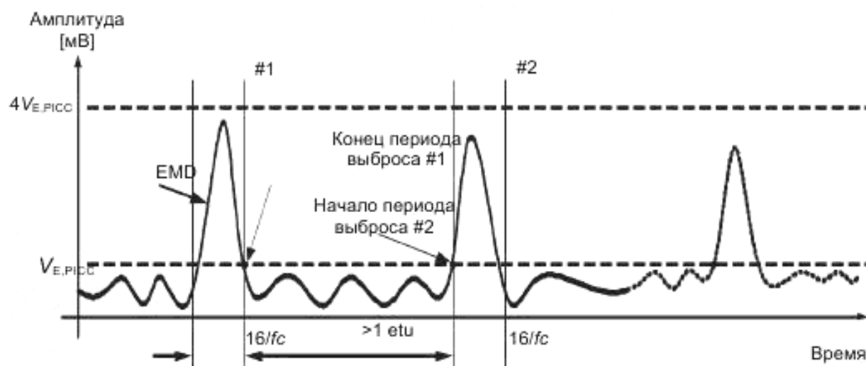
Рисунок 22 – Допустимые выбросы EMD
