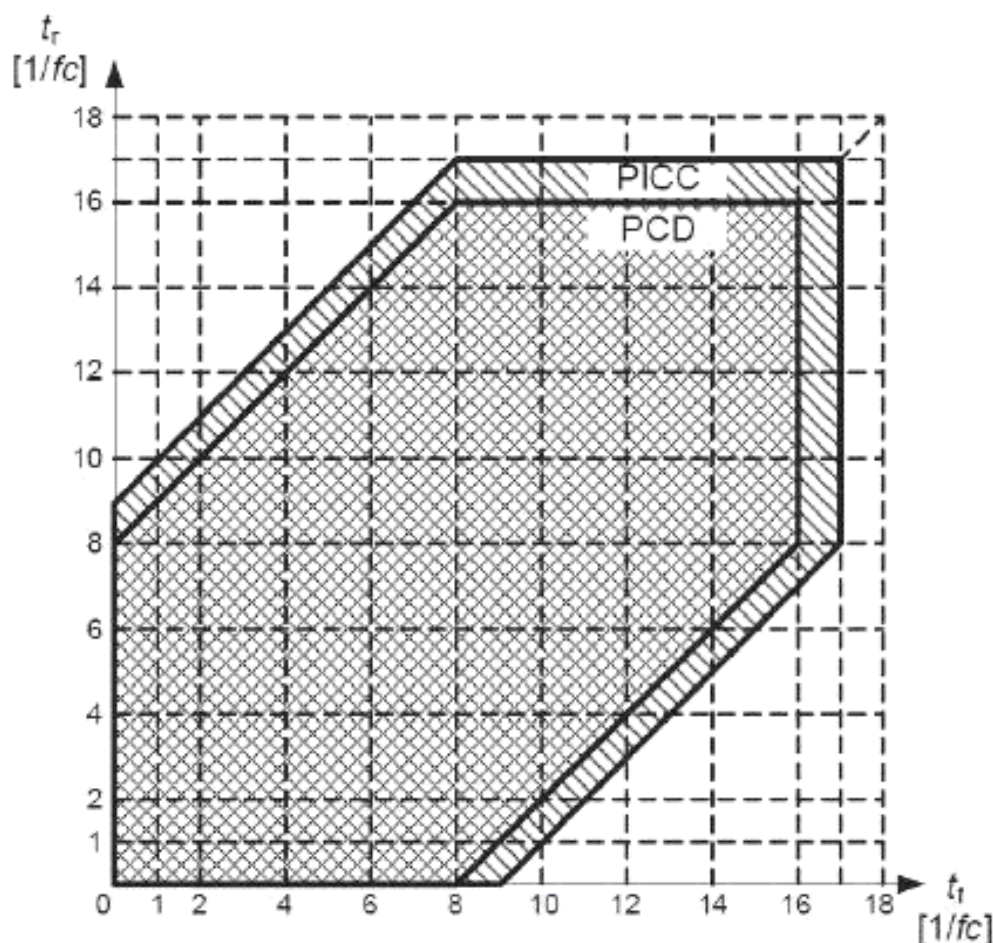
Рисунок 18– Параметры синхронизации модулированного колебательного сигнала типа В
