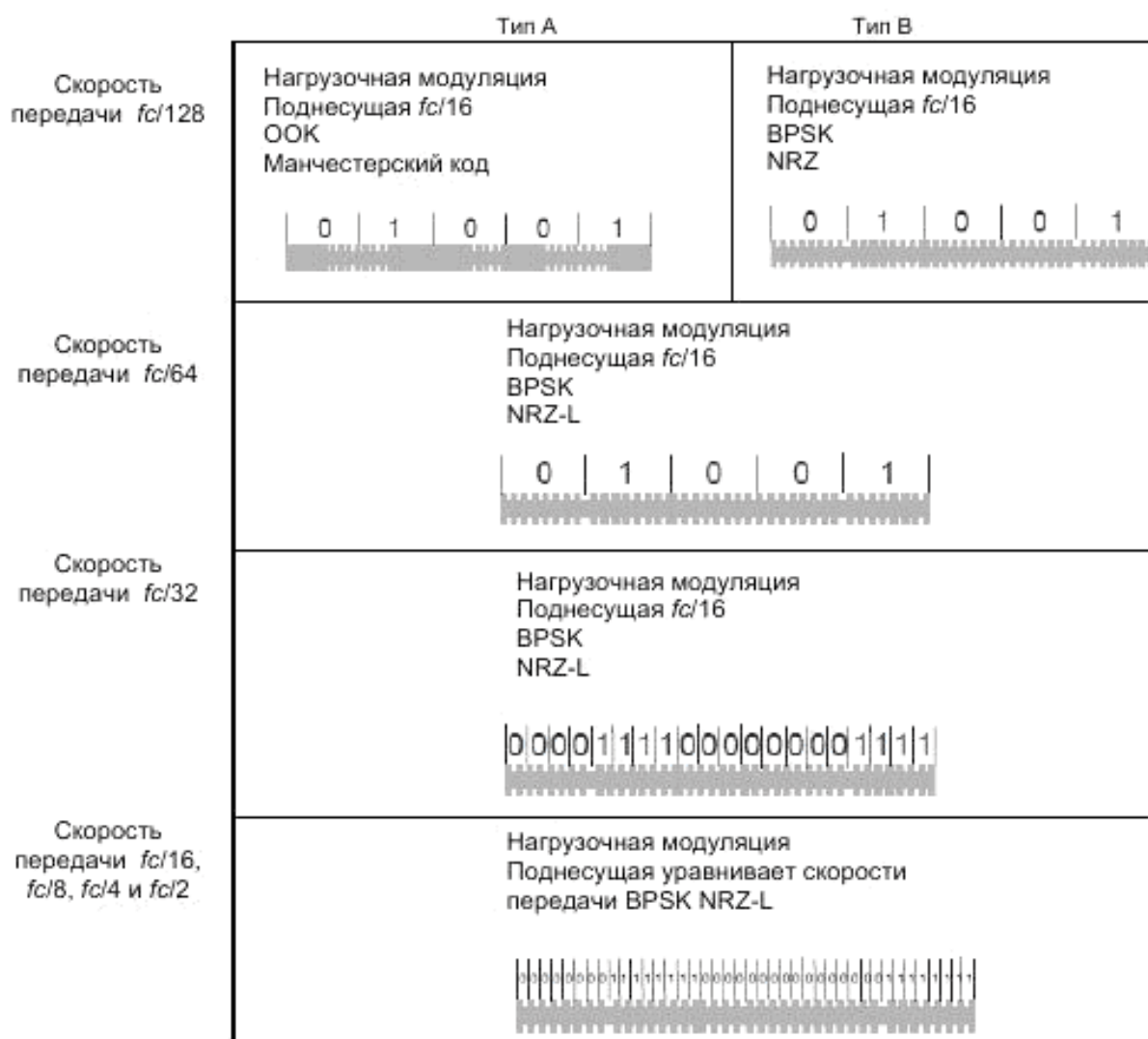
Рисунок 2 – Сигналы передачи от PICC к PCD для интерфейсов типа А и типа В (пример) (Измененная редакция, Изм. А3:2012).
