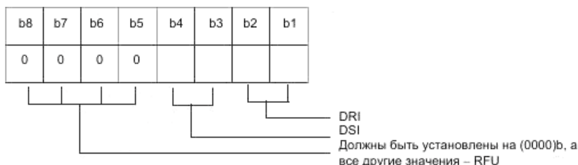
Рисунок 12 – Кодирование PPS1
