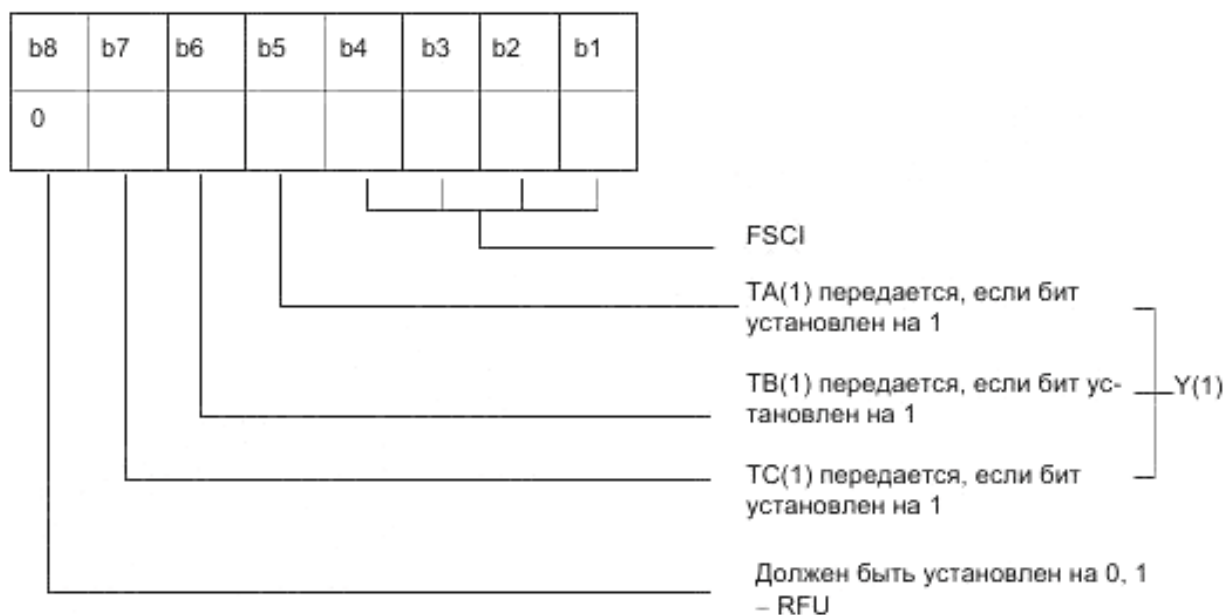
Рисунок 5 – Кодирование байта формата
