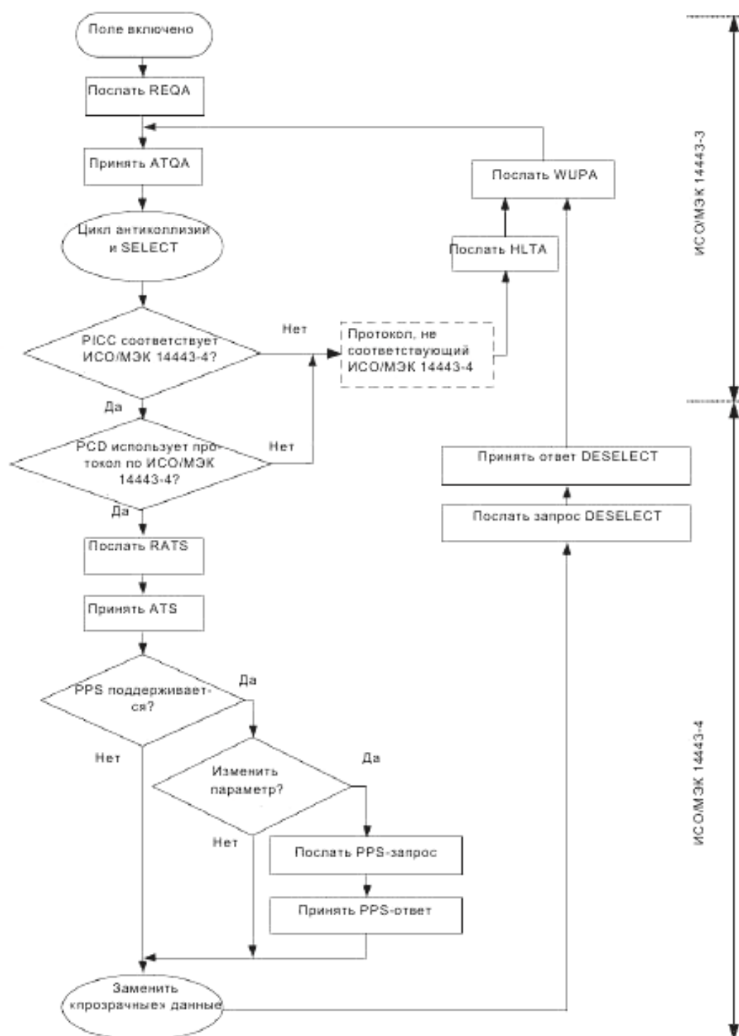
Рисунок 1 – Активация PICC типа A с помощью PCD
