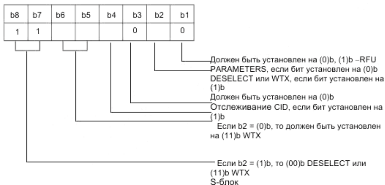
Рисунок 17 – Кодирование S-блока PCB
