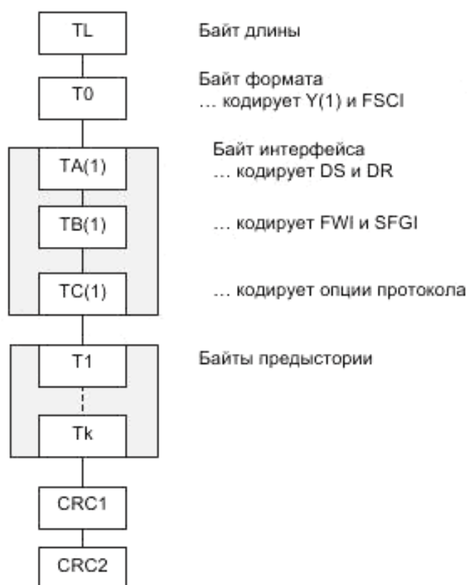
Рисунок 4 – Структура ATS
