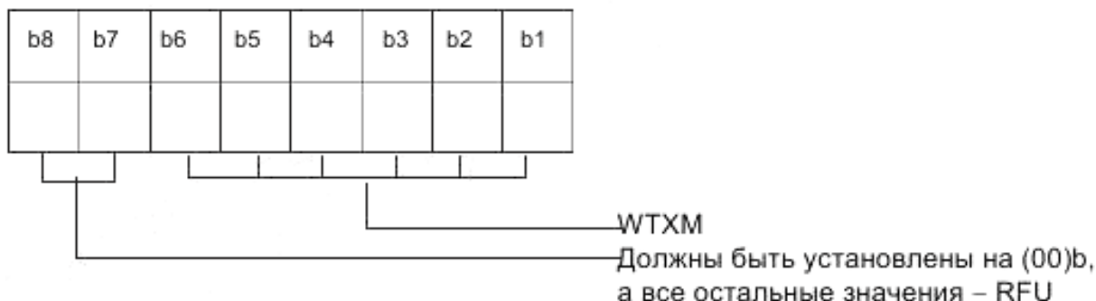
Рисунок 21 – Кодирование INF при запросе S(WTX)
