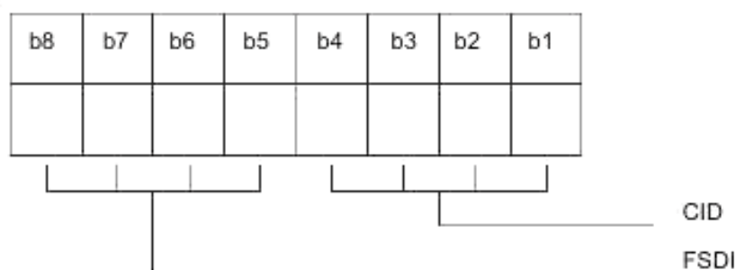
Рисунок 3 – Кодирование байта параметра RATS
