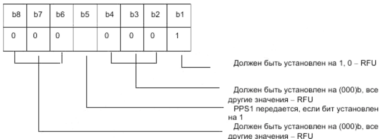
Рисунок 11 – Кодирование PPS0
