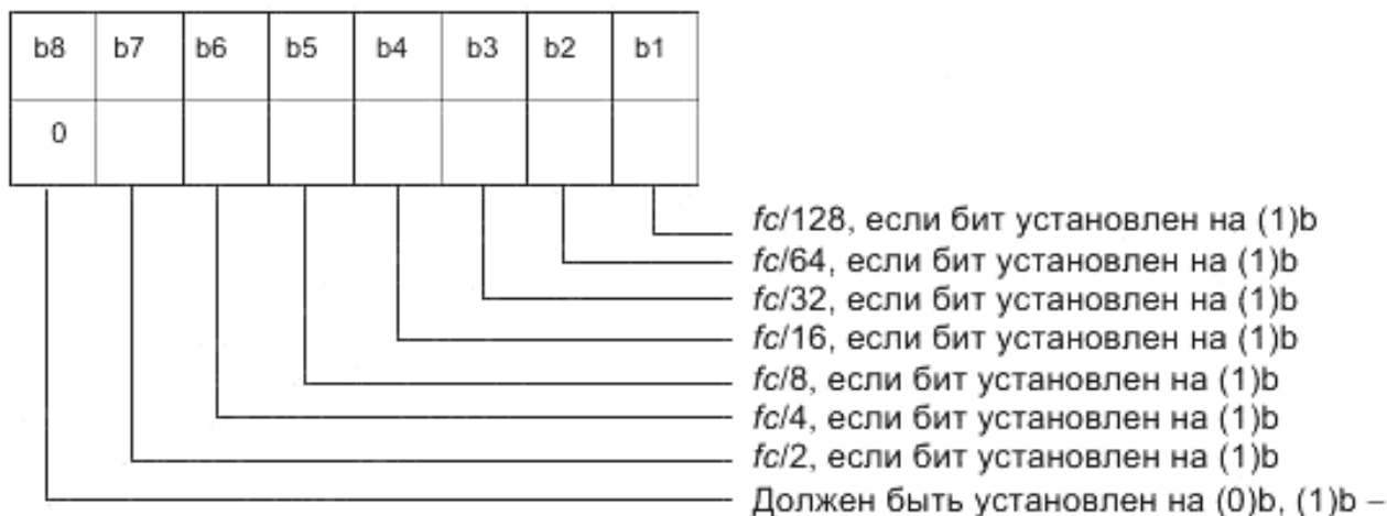
Рисунок 23 – Кодирование скоростей передачи
