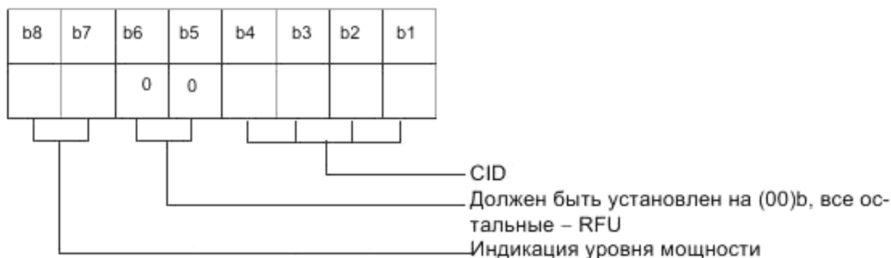
Рисунок 18 – Кодирование идентификатора карты
