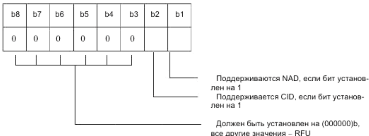
Рисунок 8 – Кодирование байта интерфейса TC(1)
