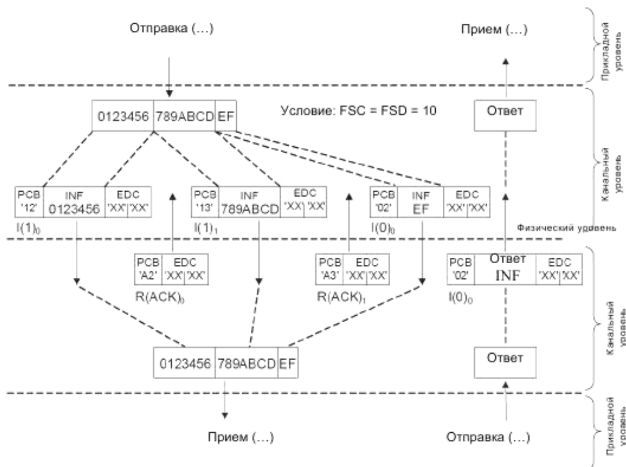
Рисунок 22 – Сцепление
