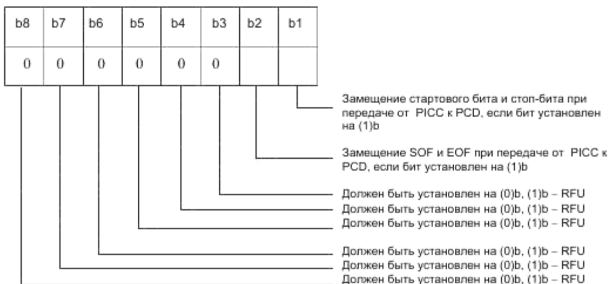
Рисунок 24 – Опции кадровой синхронизации
