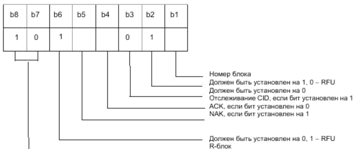
Рисунок 16 – Кодирование R-блока PCB
