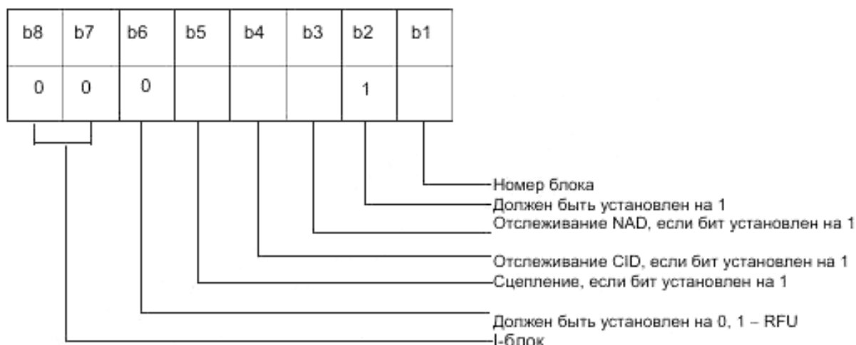
Рисунок 15 – Кодирование I-блока PCB
