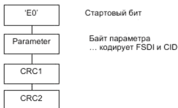
Рисунок 2 – Запрос для Ответа на Выбор
