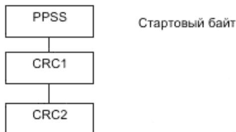
Рисунок 13 – Ответ на выбор протокола и параметров
