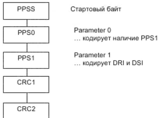
Рисунок 9 – Запрос выбора протокола и параметров
