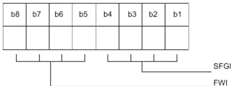
Рисунок 7 – Кодирование байта интерфейса TB(1)
