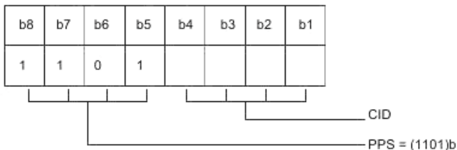
Рисунок 10 – Кодирование PPSS
