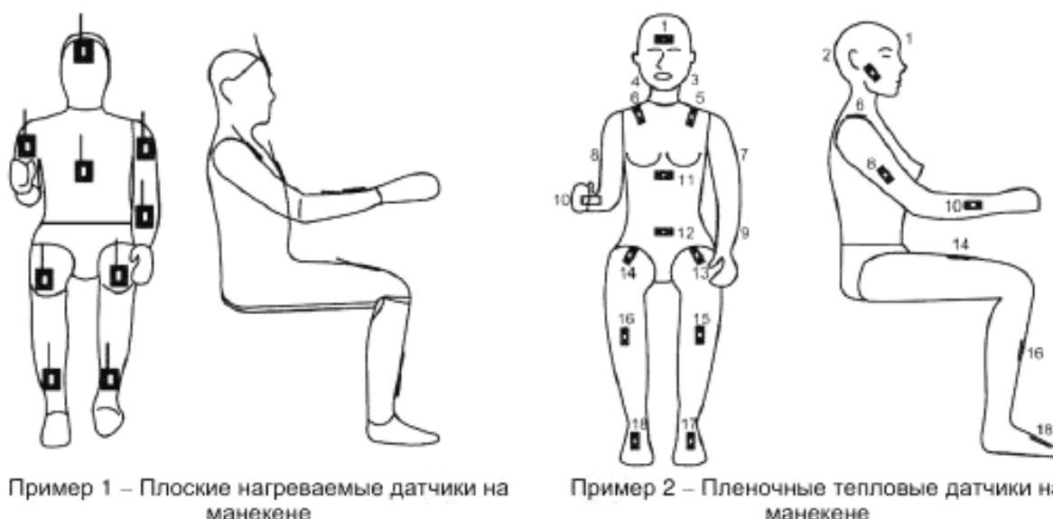
Рисунок А.2 – Примеры установки датчиков для измерения t_{\text{ср}} с использованием нескольких отдельных нагреваемых датчиков, прикрепленных к манекену или реальному человеку
