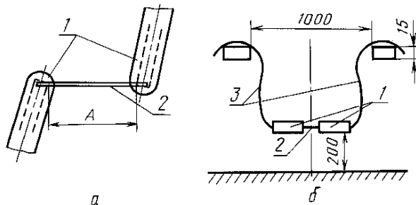
1 — электрододержатель; 2 — стержень; 3 — сварочный кабель
