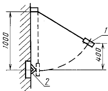
1 — электрододержатель; 2 — уголок
