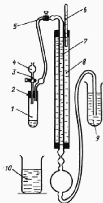
1 — реакционная пробирка; 2 — резиновая пробка с отводной трубкой и капельной воронкой; 3 — метка на капельной воронке; 4 — капельная воронка; 5 — трехходовой кран; 6 — термометр; 7 — газосборная бюретка; 8 — водяная рубашка; 9 — уравнительная склянка; 10 — водяная баня
