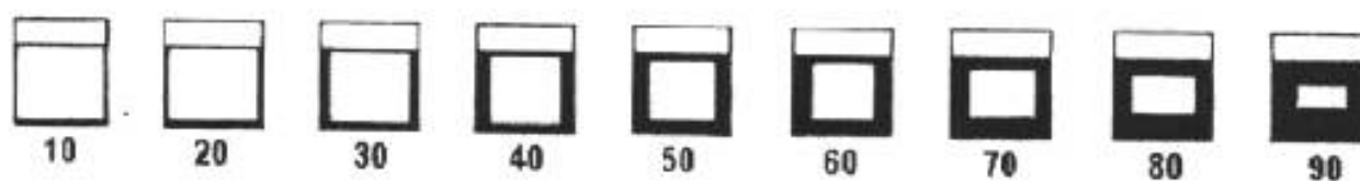
В - Руководство для оценки внешнего вида излома
