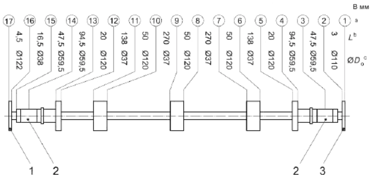
1 – ротор в осевом АМП; 2 – ротор в радиальном АМП; 3 – ротор двигателя; а – точки узлов колебаний ротора; б – длина элемента ротора L ; с – диаметр элемента ротора D_0
