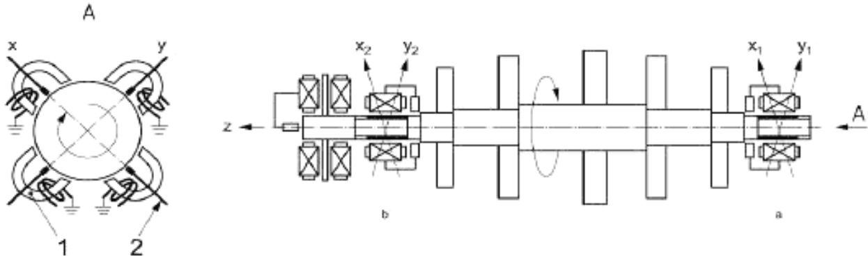
1 – АМП; 2 – датчик перемещения; a – сторона 1; b – сторона 2 Рисунок 2 – Система «ротор – АМП»
