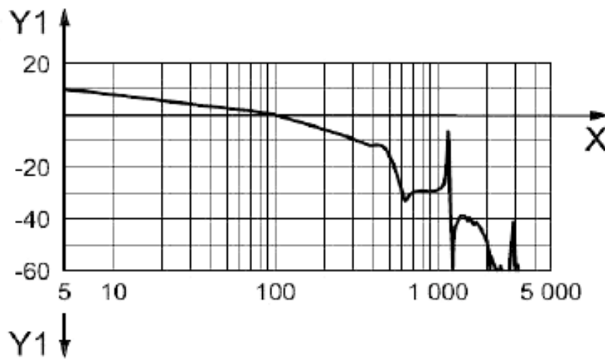
b) Управление «кососимметричными» модами X – частота, Гц; Y1 – модуль, дБ; Y2 – фаза, в градусах Рисунок С.2 (окончание)
