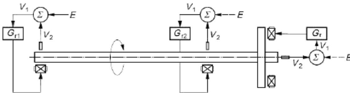
Рисунок A.5 – Раздельное управление АМП
