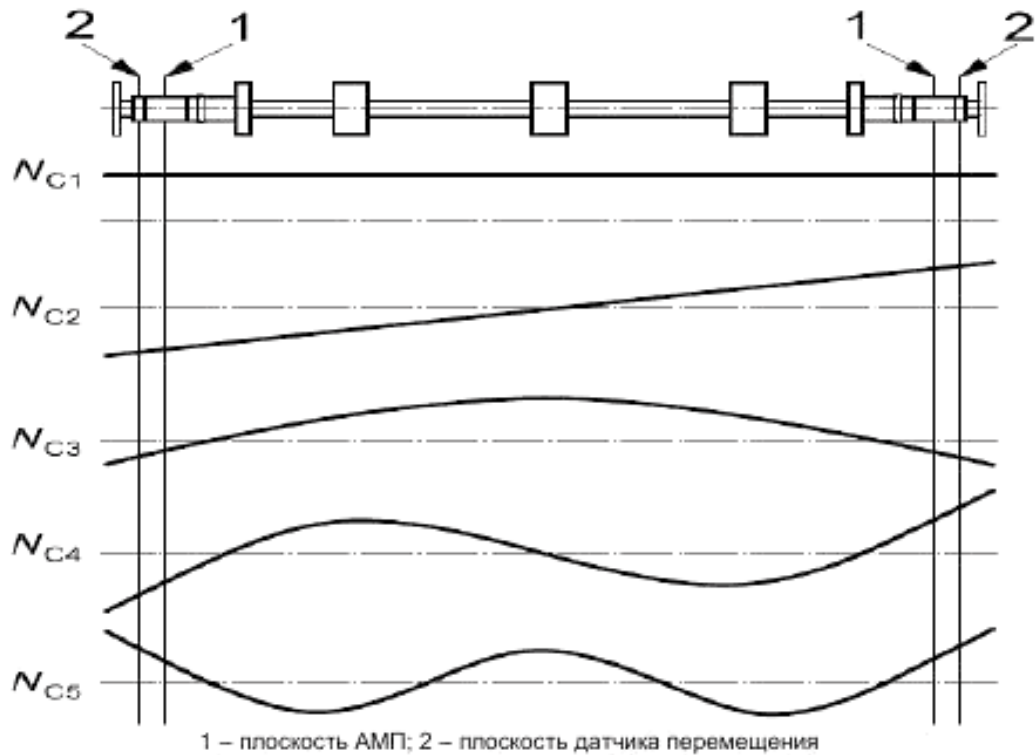
Рисунок А.3 – Собственные моды и собственные частоты N_{C1} гибкого ротора
