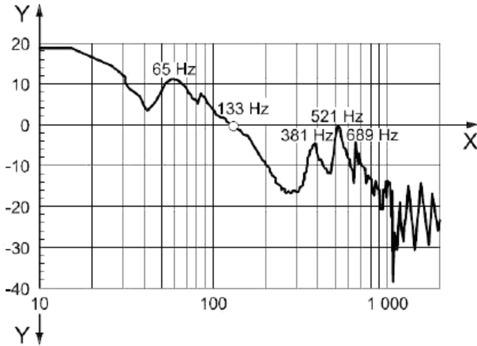
Рисунок В.2 – Диаграмма Бодэ типичной передаточной функции разомкнутой цепи G_o
