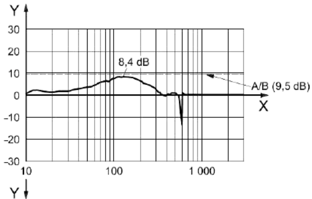
a) Управление «симметричными» модами
