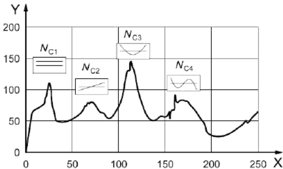
Рисунок А.10 – Изменения вибрации с изменением частоты вращения ротора
