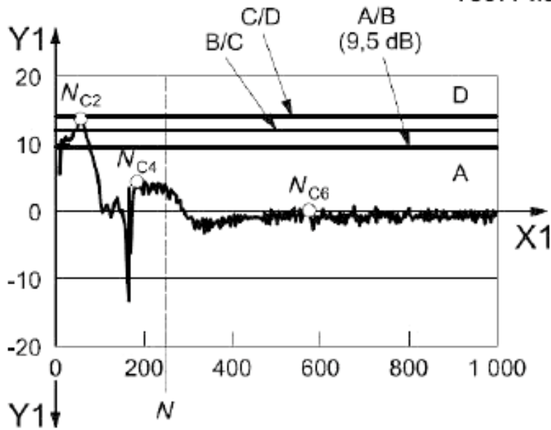
d) Функция чувствительности G_y
