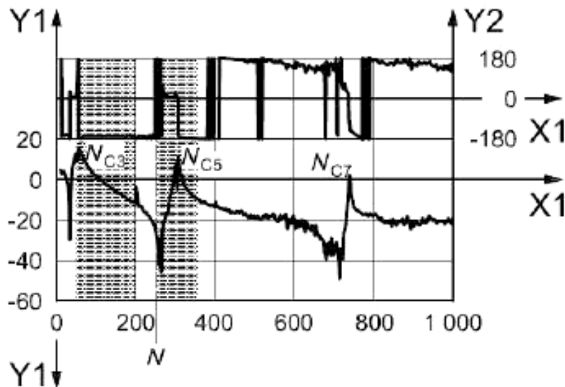
a) Диаграмма Бode передаточной функции разомкнутой цепи G_d
