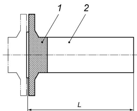
д) Фланцевое соединение
