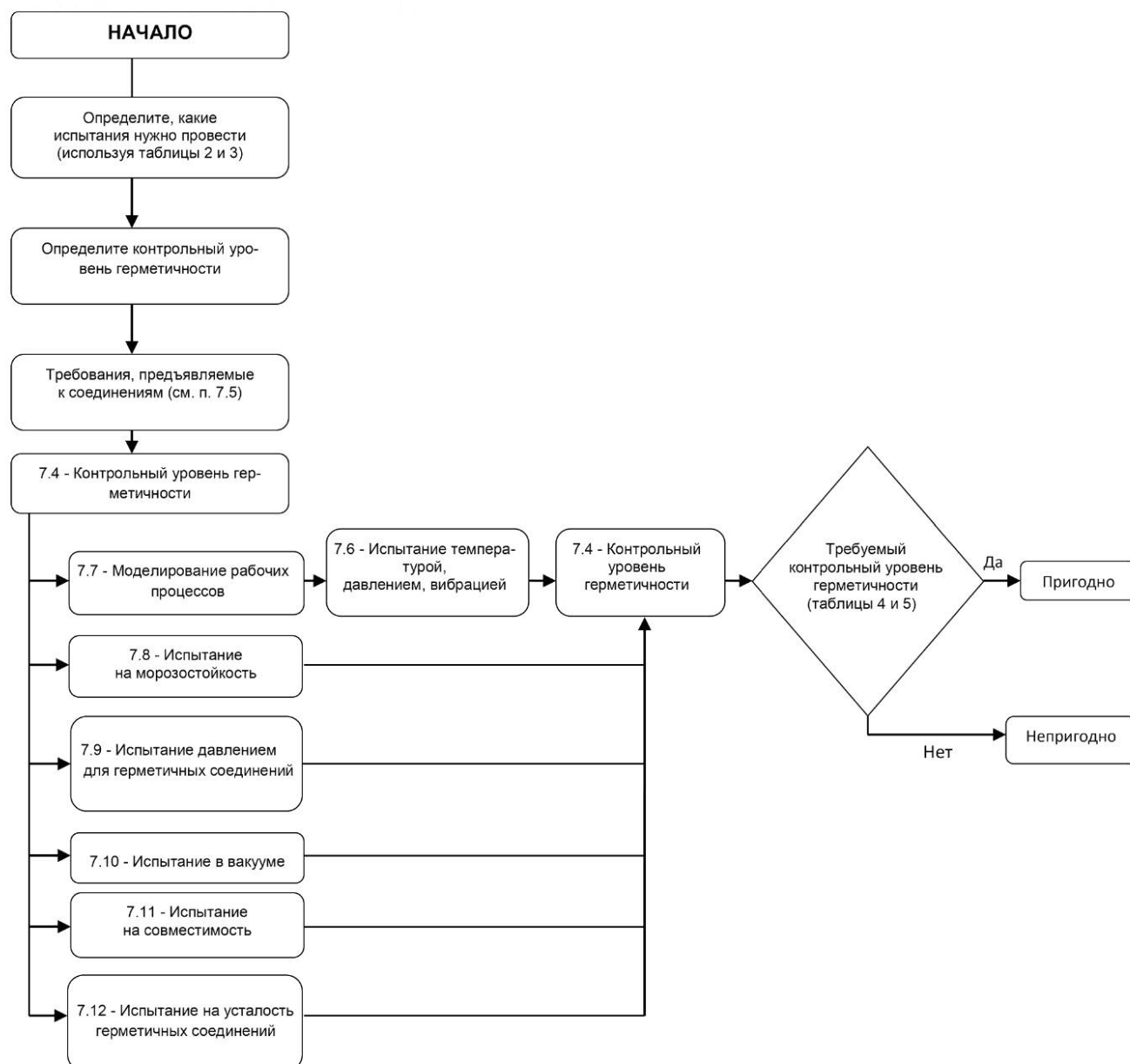
Рисунок 2 — Последовательность испытаний
