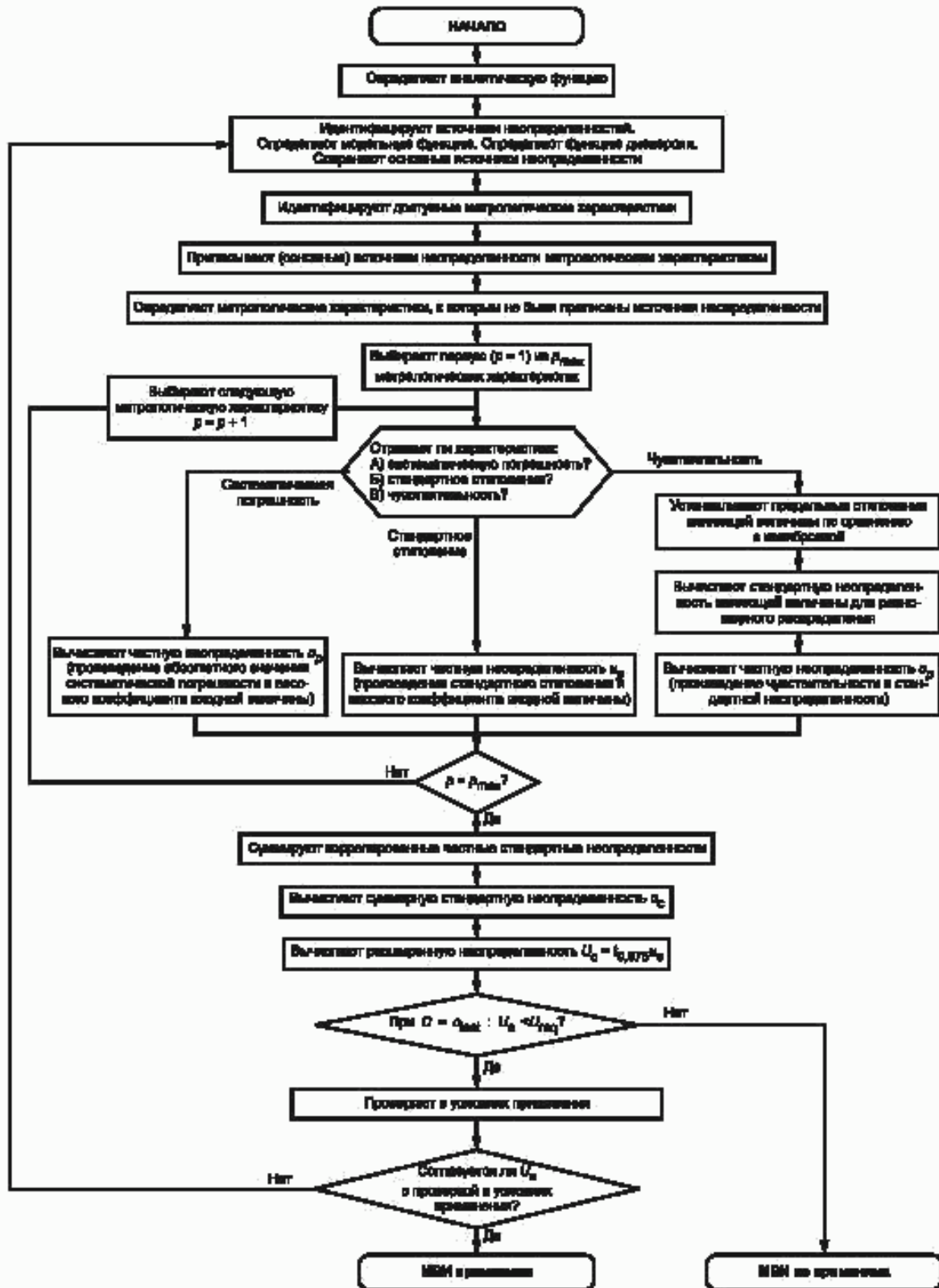
Рисунок 1 — Блок-схема для оценки пригодности МВИ для использования
