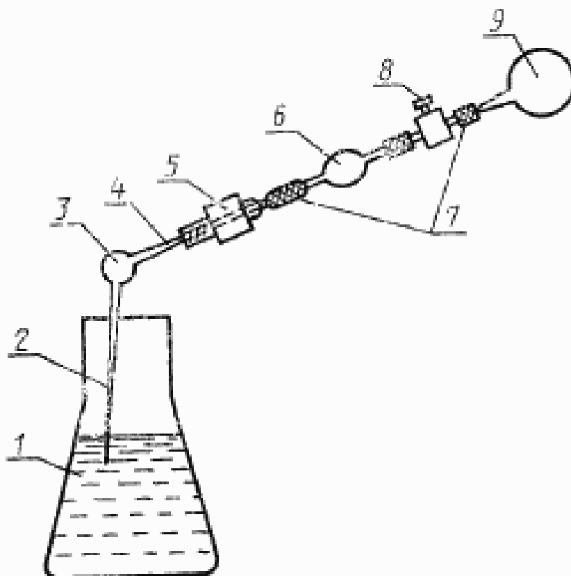
1—колба с меланжем; 2, 4—капиллярные концы ампулы; 3—ампула; 5—фторопластовый мундштук; 6—соединяющий индикатор; 7—гибный шланг; 8—вентиль; 9—резиновая груша
