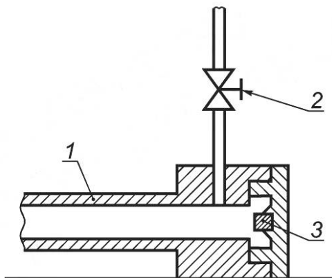
1 — соединительная трубка; 2 — запорный клапан; 3 — испытуемый образец
