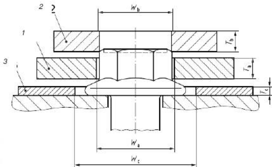
1 — калибр А; 2 — калибр В; 3 — калибр С W_{A, \min} = e_{\text{теор}} ; W_{B, \max} = e_{\min} - 0,01 \text{ мм} ; T_{A, \max} = k_{A, \min}
