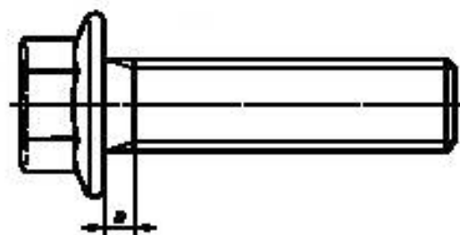
Рисунок 4 — Болт с шестигранной головкой с фланцем с резьбой до головки
