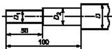
Рисунок А.1 — Форма образца
