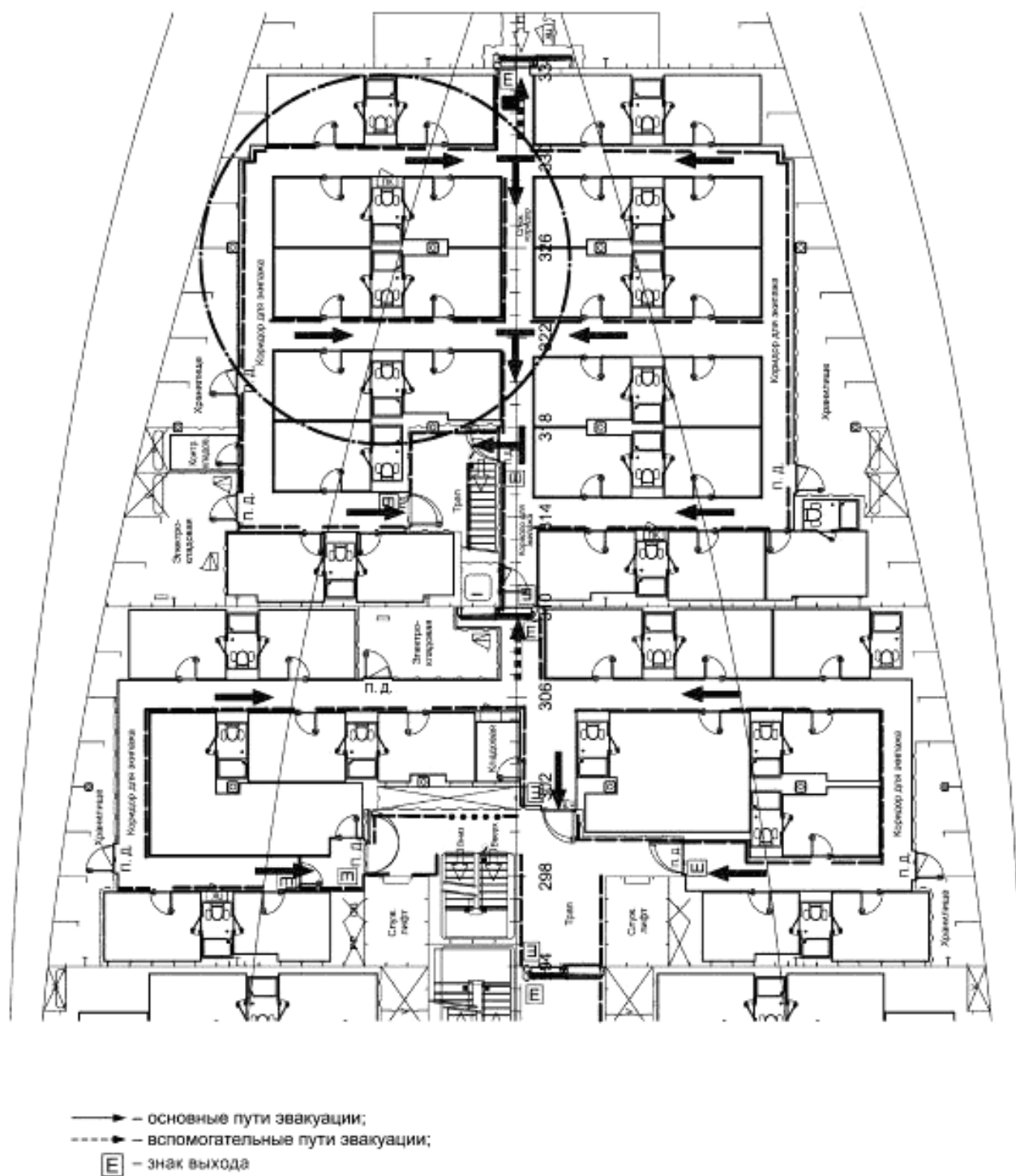
Рисунок G.5 — Пример, поясняющий 6.2.1. Типичное расположение элементов системы НРО, при котором исключается возможность образования «петель» вокруг одного жилого помещения
