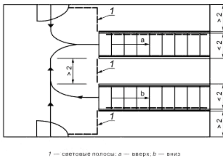
Рисунок F.2 — Расположение световых полос в выгородках трапа
