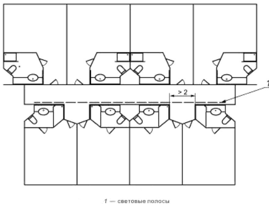
Рисунок F.1 — Расположение световых полос для коридорной ниши
