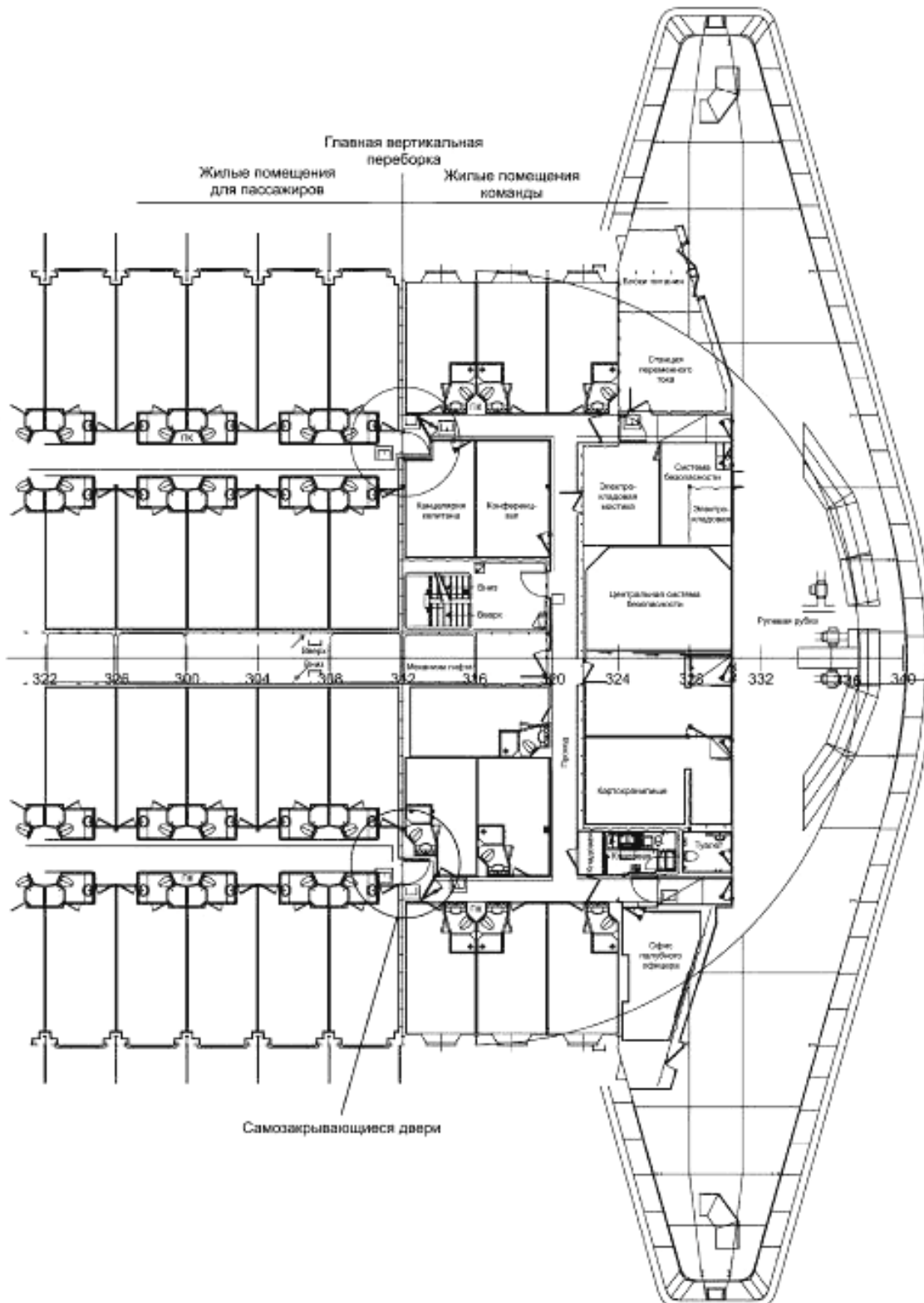
Рисунок G.2 — Пример, поясняющий 6.1.6. Расположение электрических и ФЛ-систем НРО на одной палубе: фотолюминесцентное освещение, установленное в жилых помещениях экипажа, сменяется на электрическое в жилых помещениях для пассажиров
