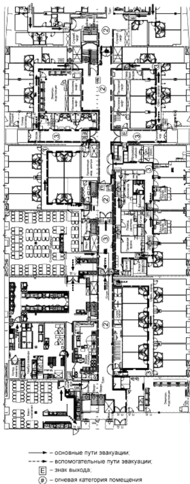
Рисунок G.9 — Пример, поясняющий 6.5.5. Расположение двух знаков выхода на двухстворчатых дверях в пределах выгородки трапа
