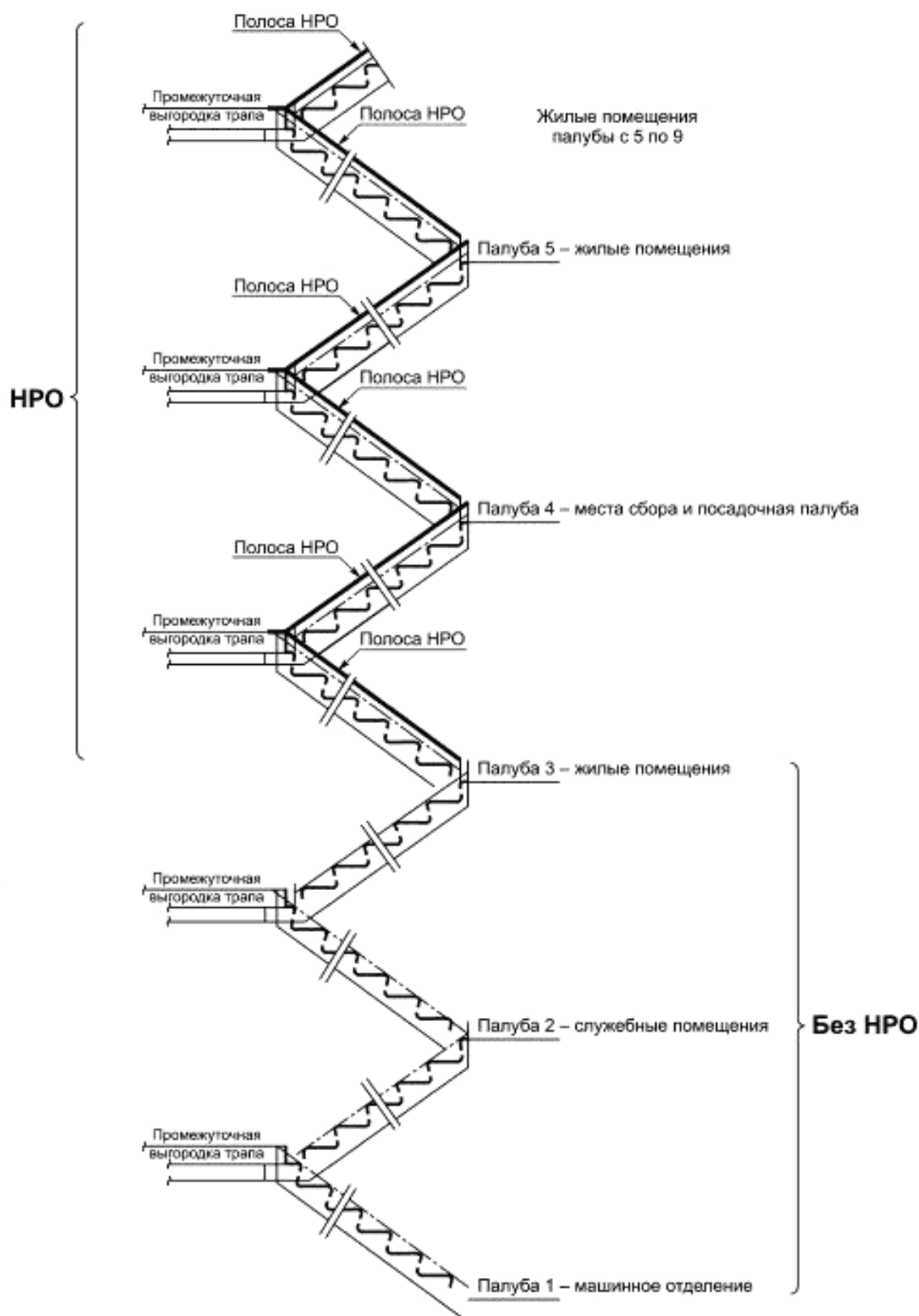
Рисунок G.7 — Пример, поясняющий 6.4.3. Единый трап, соединяющий машинное отделение, служебные и жилые помещения, где установлена система НРО и где она не установлена
