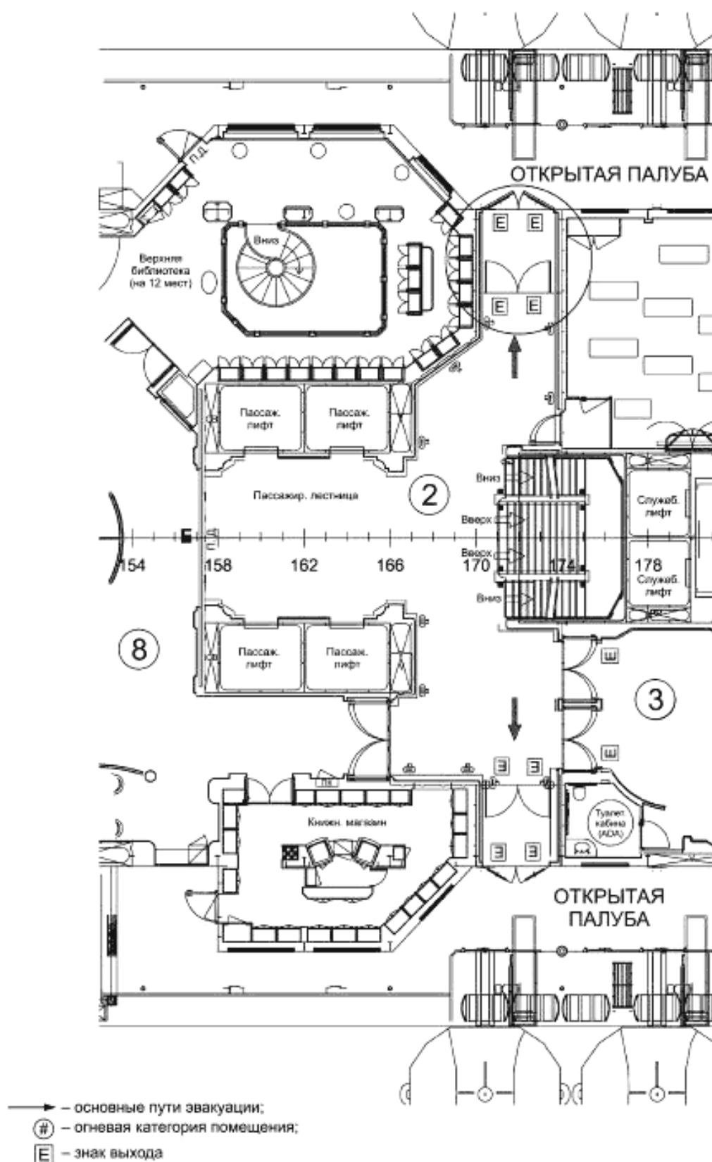
Рисунок G.8 — Пример, поясняющий 6.5.5. Расположение двух знаков выхода на двухстворчатых дверях, ведущих на открытую палубу
