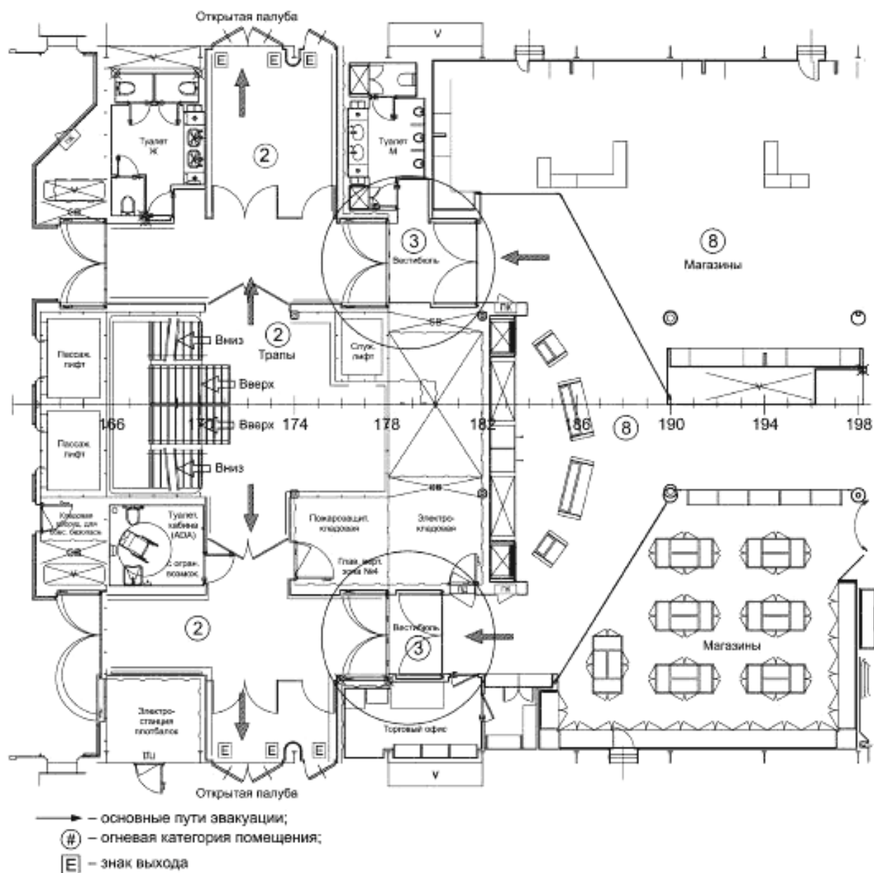
Рисунок G.3 — Пример, поясняющий 6.1.3. Небольшой изолированный вестибюль 3-й огневой категории без установки системы НПО
