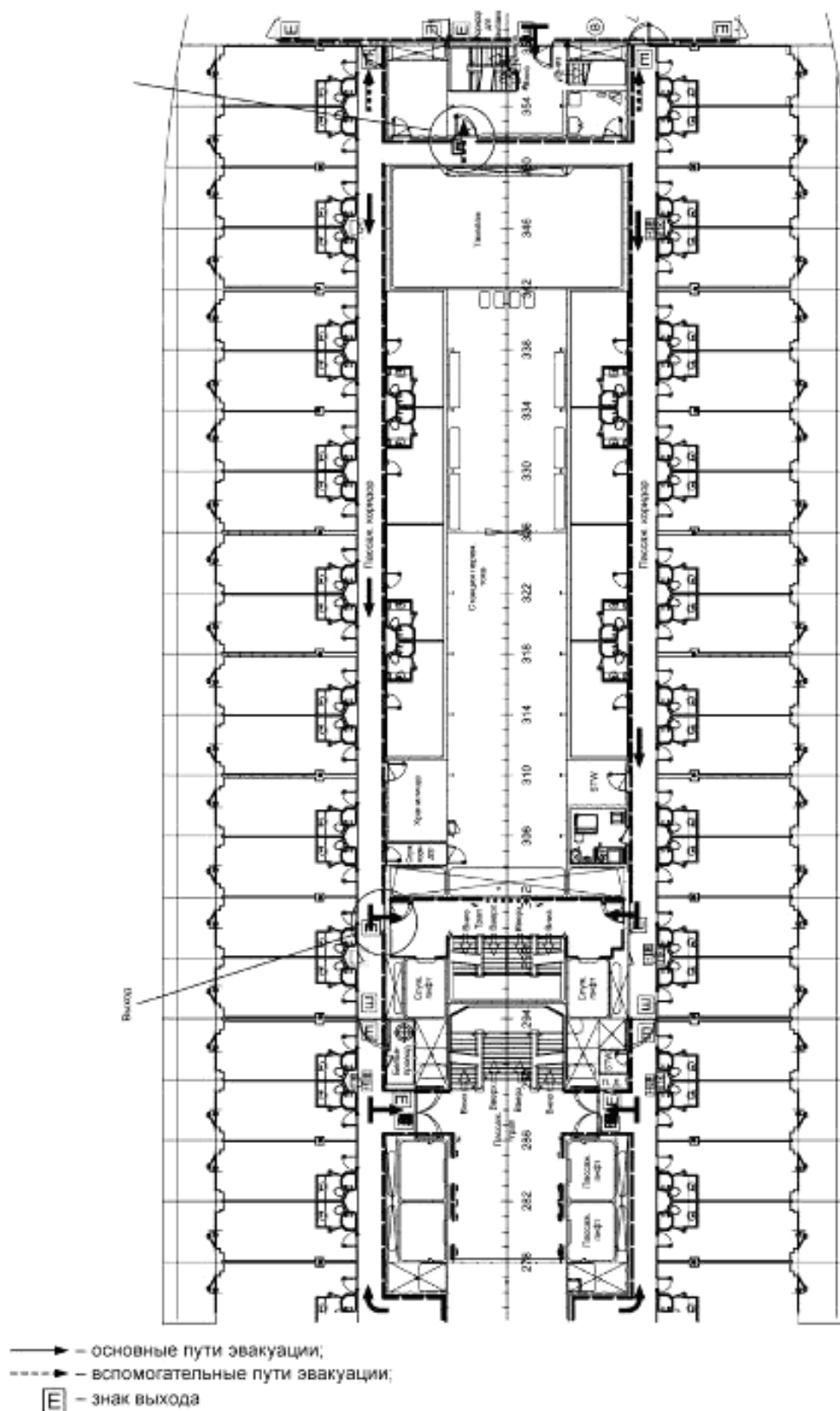
Рисунок G.6 — Пример, поясняющий 6.2.2. Полосы НРО расположены только на стороне коридора, где находится дверь выхода
