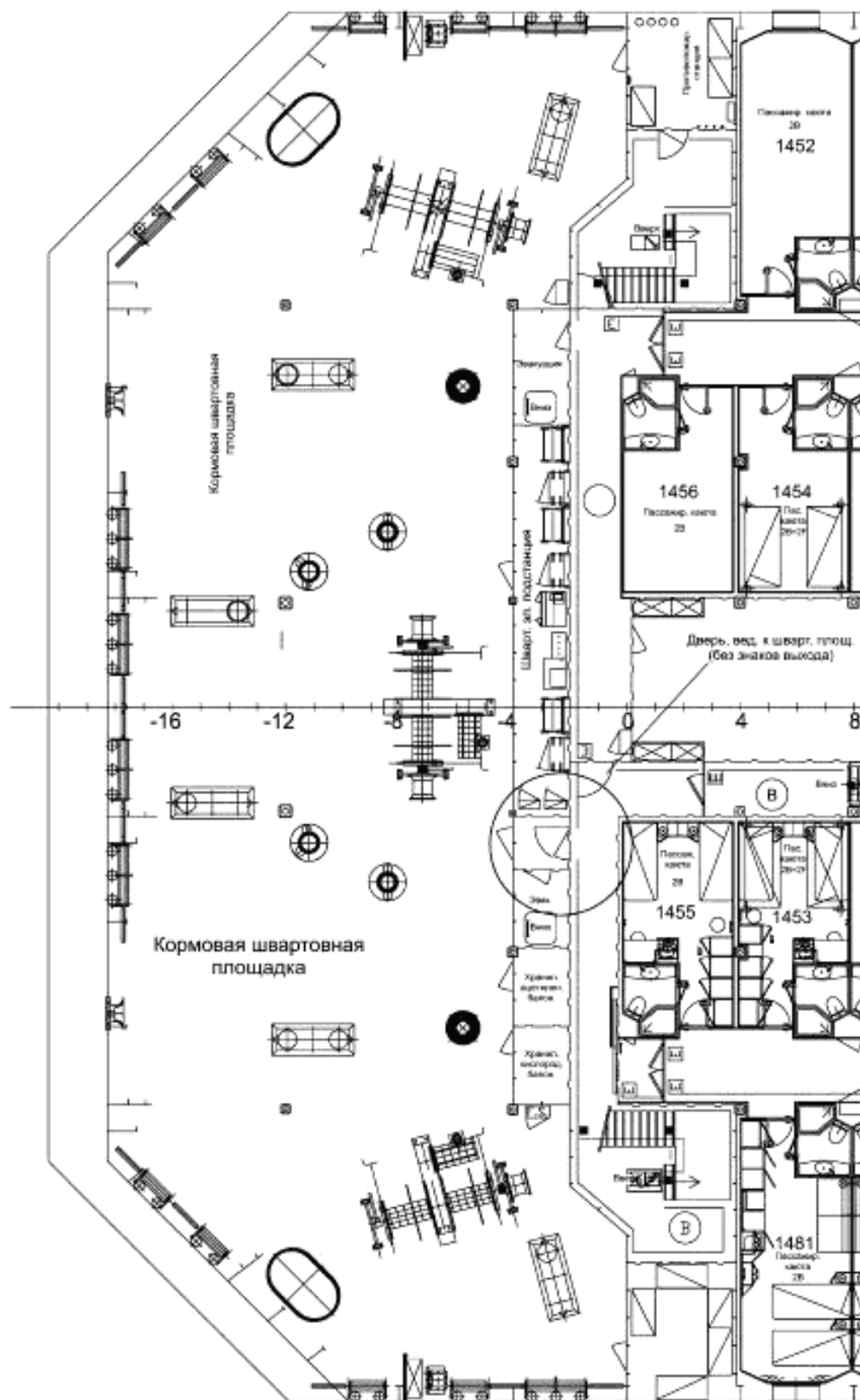
Рисунок G.10 — Пример, поясняющий 6.5.5. Расположение, когда дверь, не отмеченная знаком выхода, ведет на открытую палубу, с которой нет альтернативных эвакуационных выходов
