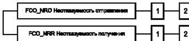
Рисунок D.1 — Декомпозиция класса FCO «Связь»
