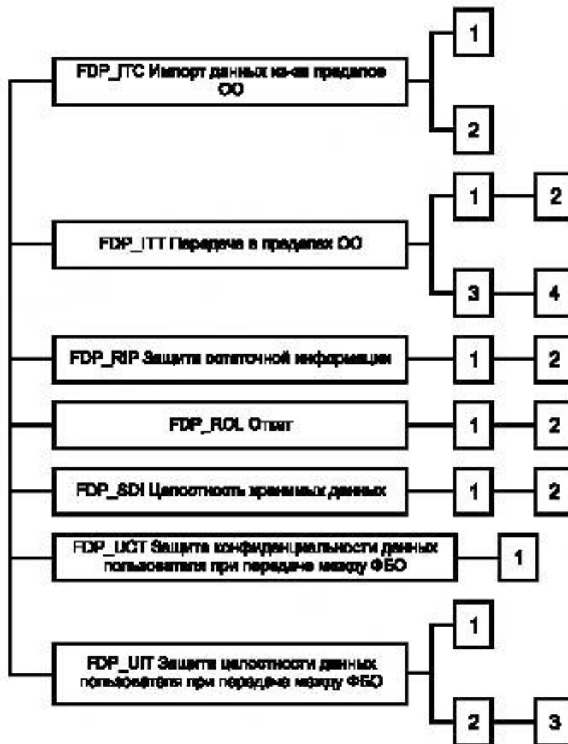
Рисунок 10 — Декомпозиция класса FDP «Защита данных пользователя» (продолжение)
