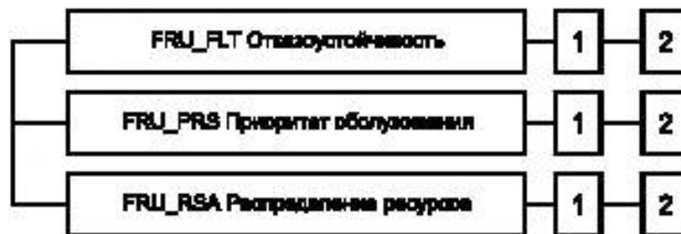
Рисунок К.1 — Декомпозиция класса FRU «Использование ресурсов»
