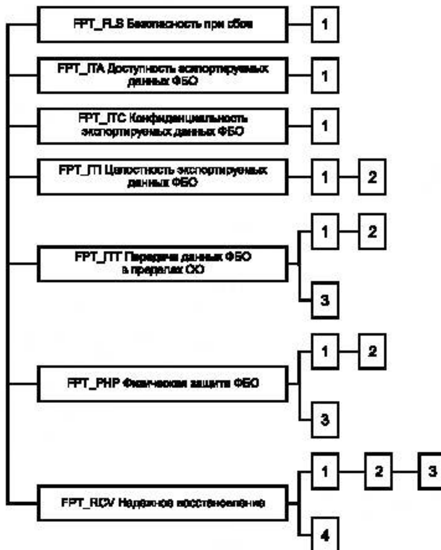
Рисунок J.1 — Декомпозиция класса FPT «Защита ФБО»
