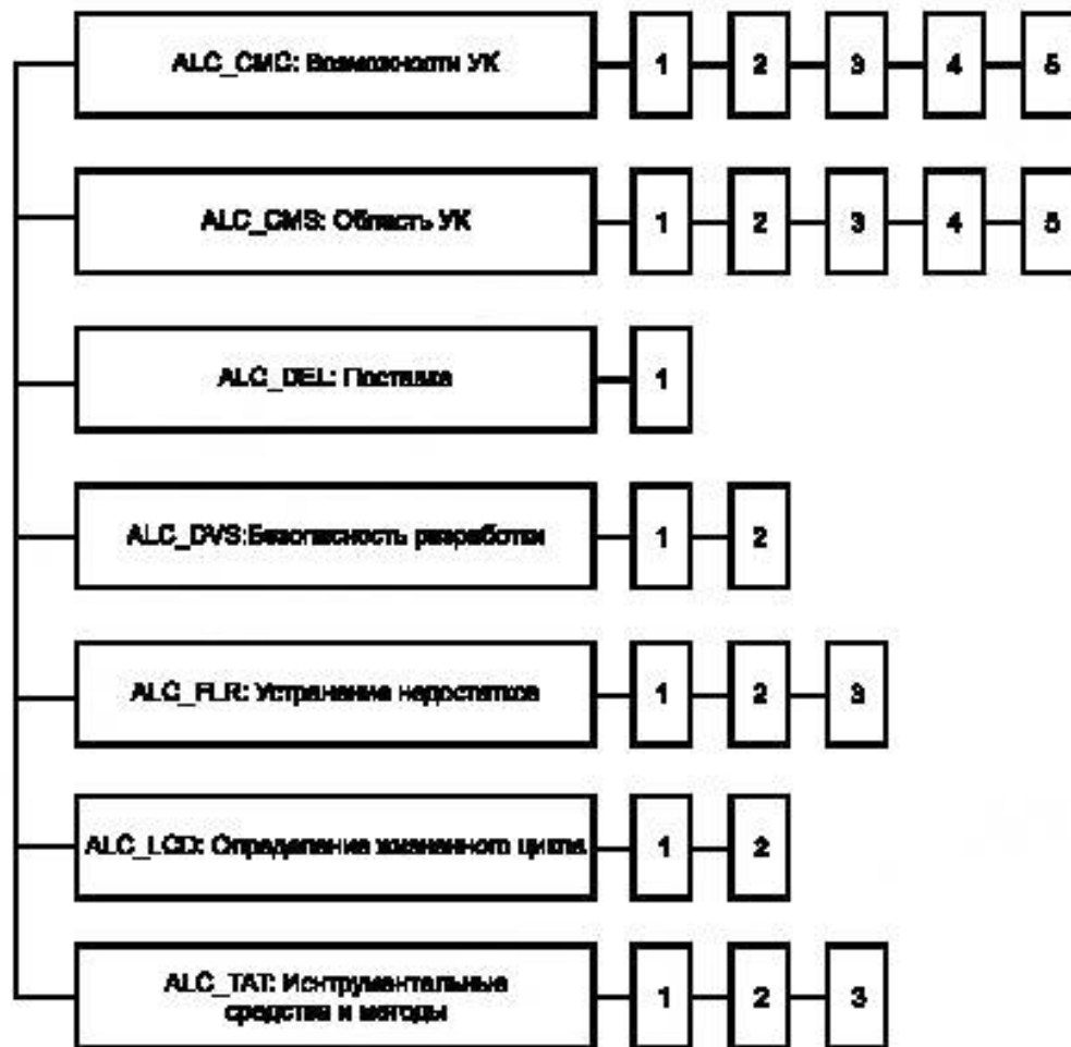
Рисунок 13 — Декомпозиция класса ALC «Поддержка жизненного цикла»
