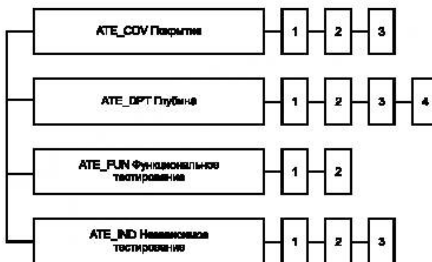
Рисунок 14 — Декомпозиция класса ATE «Тестирование»
