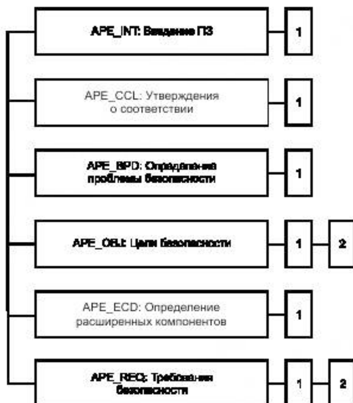
Рисунок 8 — Декомпозиция класса APE «Оценка профиля защиты»
