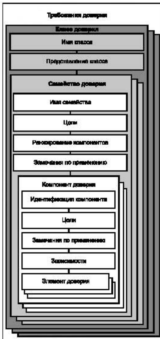
Рисунок 1 — Иерархическая структура представления требований доверия: класс-семейство-компонент-элемент.
