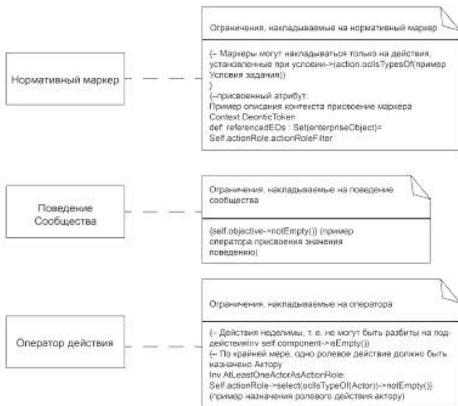
Рисунок А.2 — Понятия (концепты) описания сообщества
