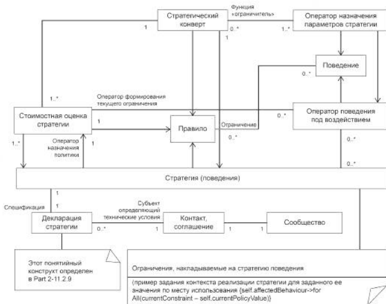
Рисунок А.4 — Понятия описания стратегий поведения
