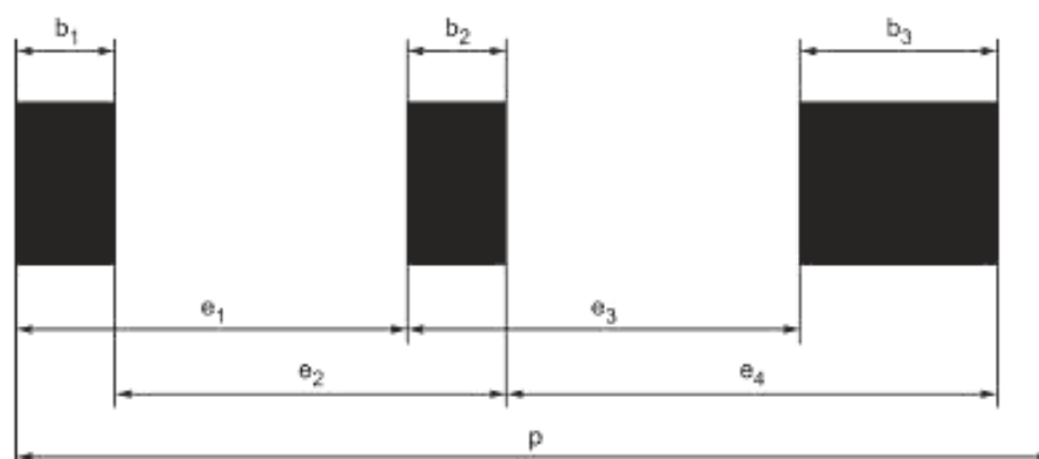
Рисунок 5 — Декодирование размеров
