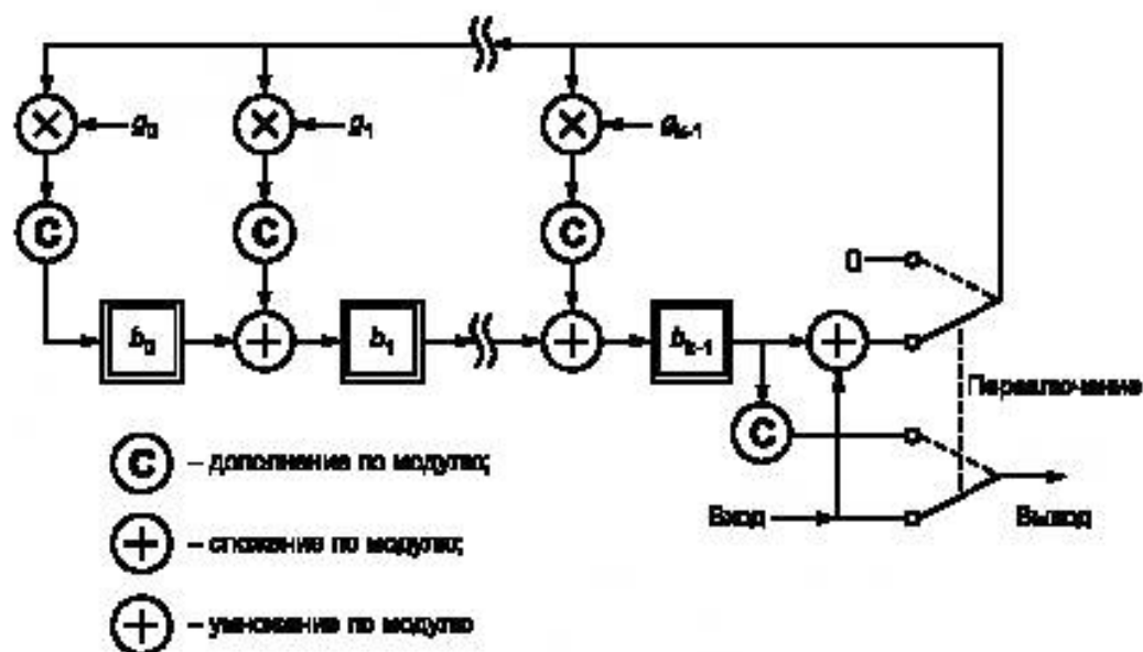
Рисунок R.1 — Схема кодирования кодовых слов коррекции ошибок
