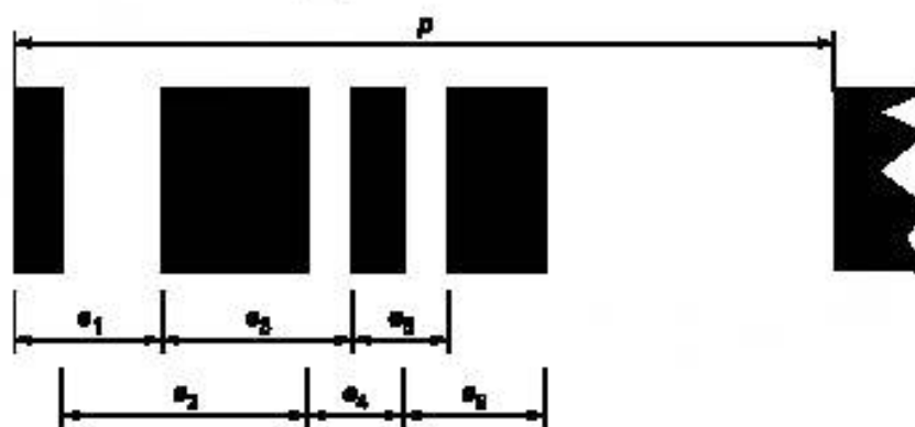
Рисунок J.1 — Размеры для декодирования
