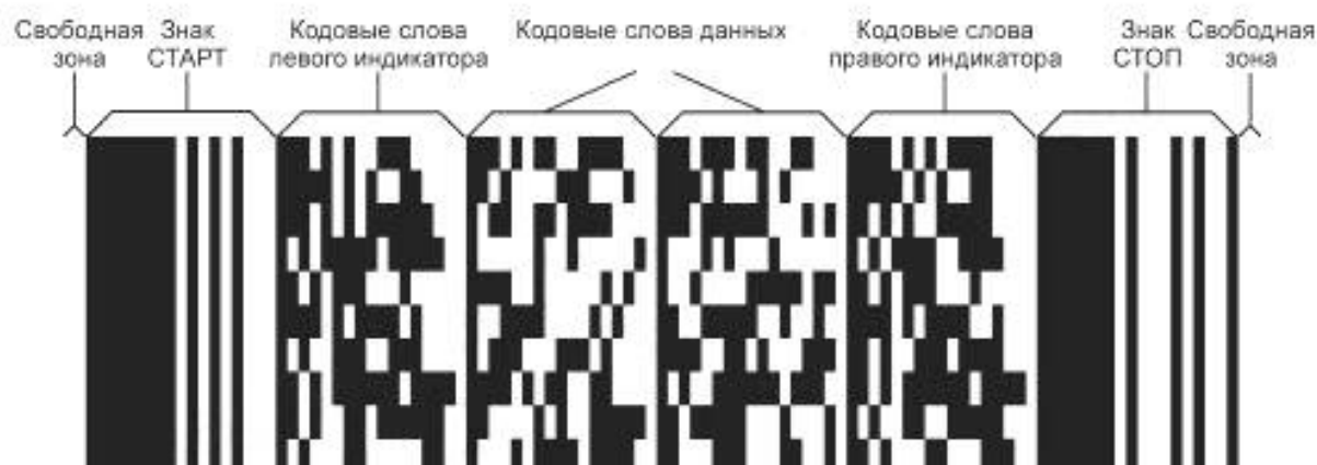
Рисунок 1 — Структура символа PDF417
