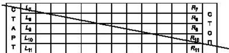
Рисунок J.2 — Схема, представляющая линию сканирования, пересекающую строки
