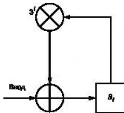
Рисунок К.1 — Делитель синдрома символа
