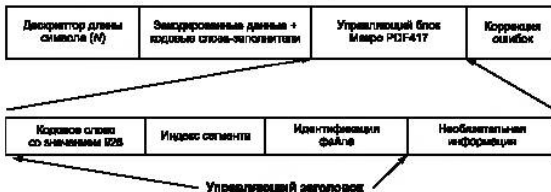
Рисунок Н.1 — Схемы символов PDF417
