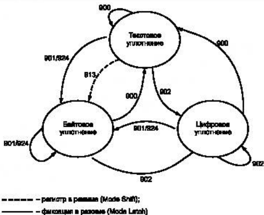
Рисунок 5 — Возможные переходы между режимами
