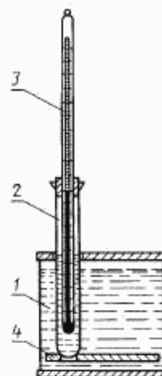
1 — масляная баня; 2 — стеклянная пробирка; 3 — термометр; 4 — металлический диск
