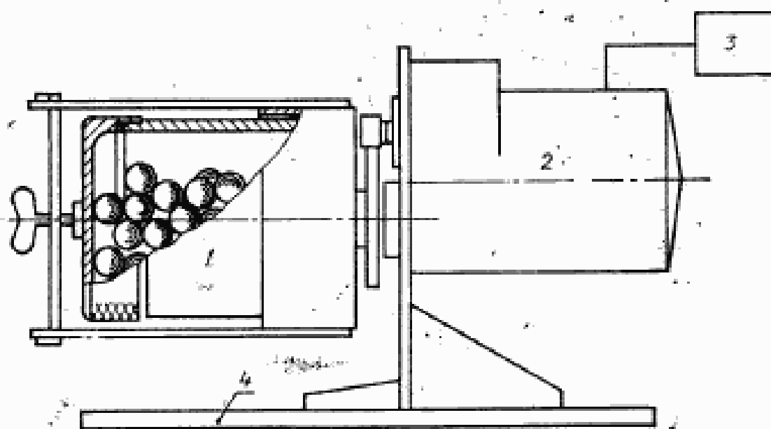
1 — барабан; 2 — мотор-редуктор; 3 — реле времени; 4 — подставка
