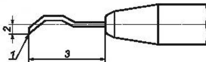
1 — наконечник инструмента; 2 — смещение; 3 — длина
