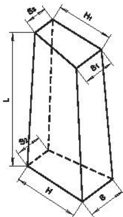
Рисунок 3 – Изделие фасонное номеров 6–9
