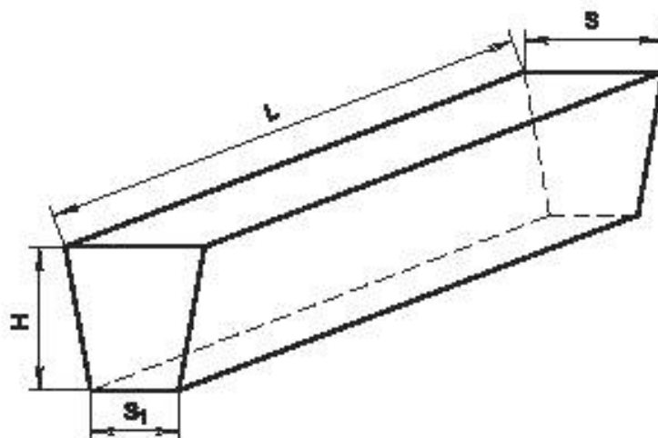
Рисунок 6 – Ребровый двусторонний клин
