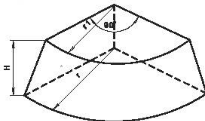
Рисунок 4 – Изделие фасонное номеров 10, 11
