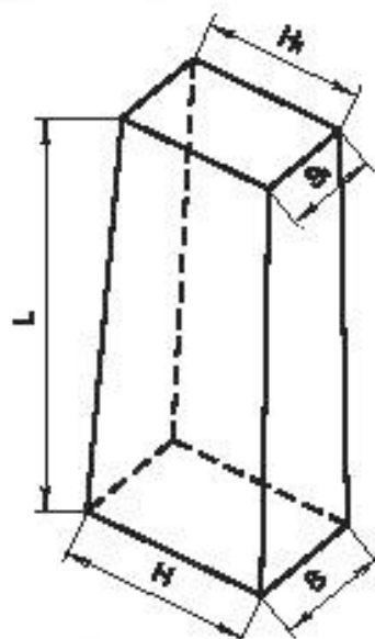
Рисунок 2 – Изделие фасонное номеров 4, 5
