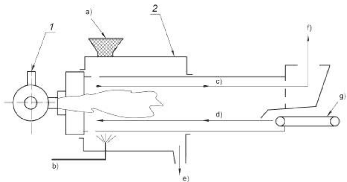
1 — горелка; 2 — сушильно-смесительный барабан для вторично используемых материалов и УАП; а) — заполнитель из вторично используемых материалов и УАП; б) — подача вяжущего; с) — направление потока газов; d) — направление движения заполнителя; е) — выход материалов, покрытых вяжущим; f) — выход газов к пылеуловителю; g) — подача холодного заводского заполнителя из натуральных материалов
