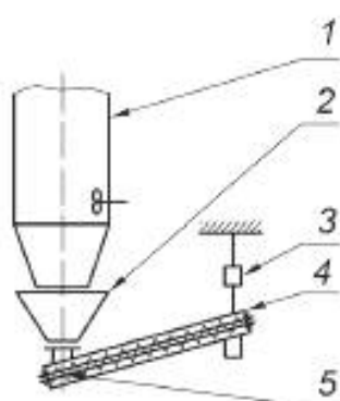
б) Непрерывного действия со шнековым питанием
