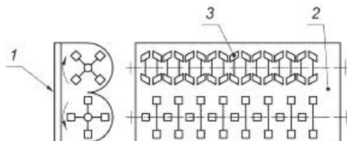
б) Двухвальный лопастной смеситель непрерывного действия
