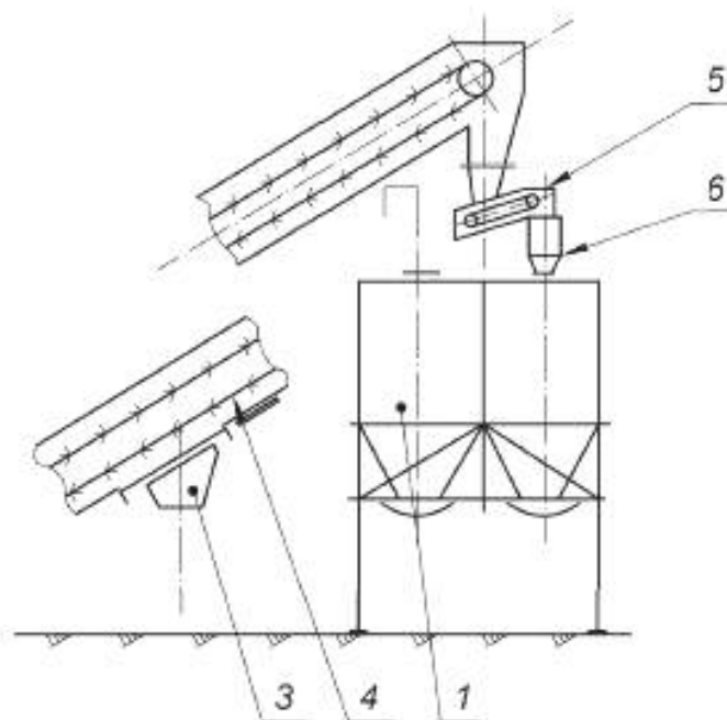
б) Со скребковым конвейером
