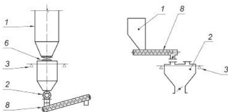
а) Циклическое действие
