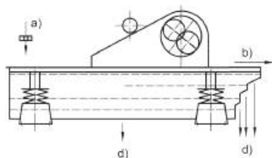
б) Вибрационный грохот с горизонтальной просеивающей поверхностью
