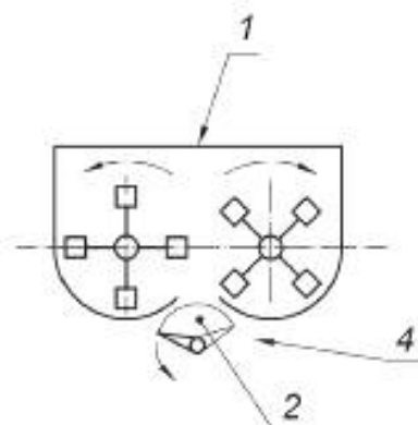
д) Двухвальный лопастной смеситель циклического действия
