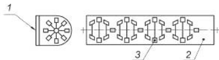
а) Одновальный лопастной смеситель непрерывного действия
