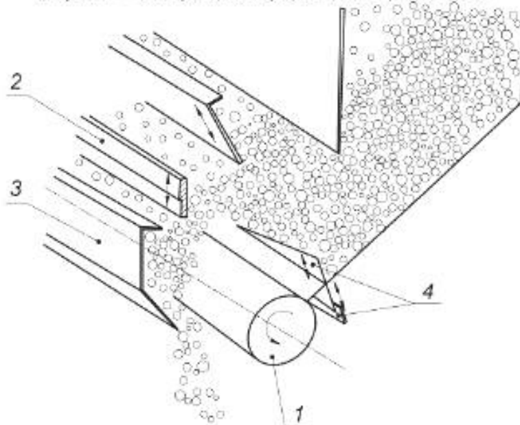
1 — подающий барабан; 2 — шибер; 3 — питатель; 4 — задвижки бункера или наклонная заслонка
