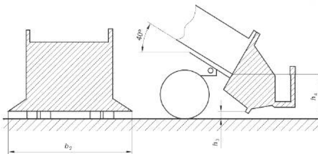
б) в рабочем положении
