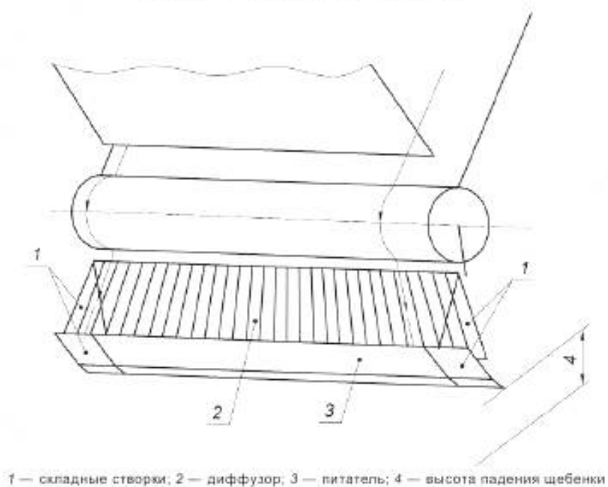
Рисунок 7 — Диффузор с питателем
