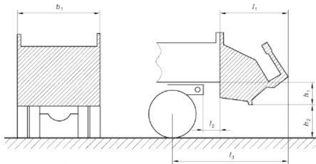
а) в транспортном положении
