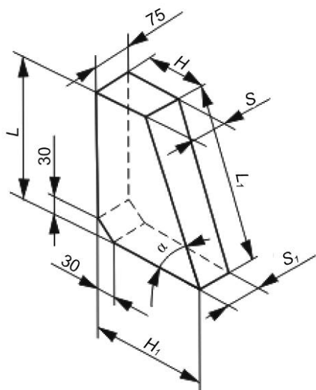
Рисунок 8 — Опорный кирпич
