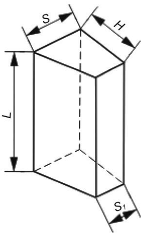
Рисунок 6 — Электродный кирпич
