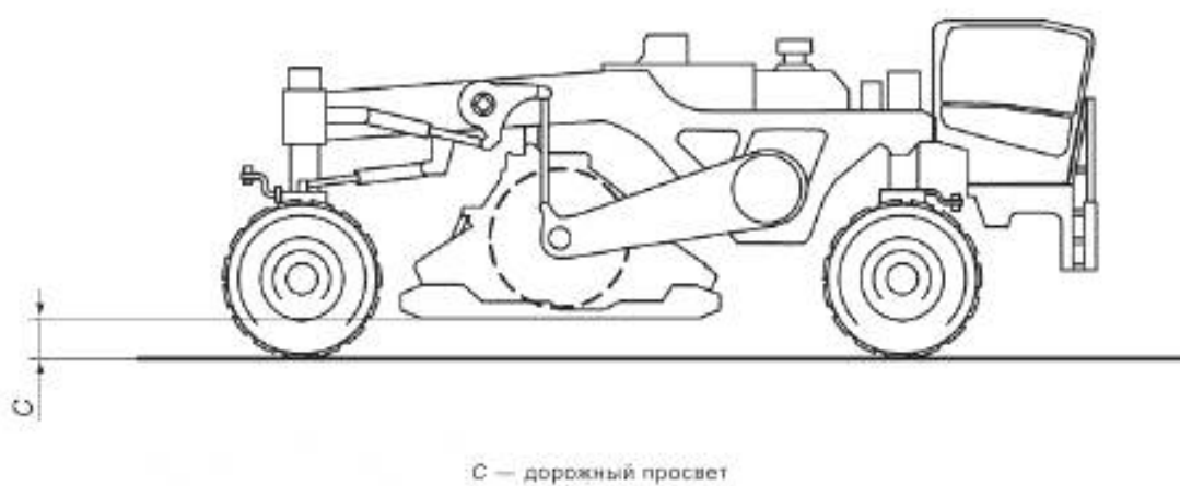
Рисунок А.13 — Дорожный просвет на примере стабилизатора грунта
