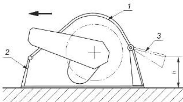
1 — корпус смесительной камеры; 2 — передняя заслонка; 3 — задняя заслонка
