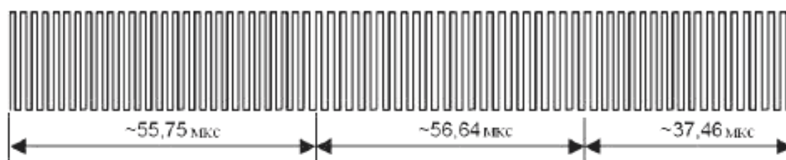
Рисунок 15 – Начало кадра при использовании двух поднесущих
