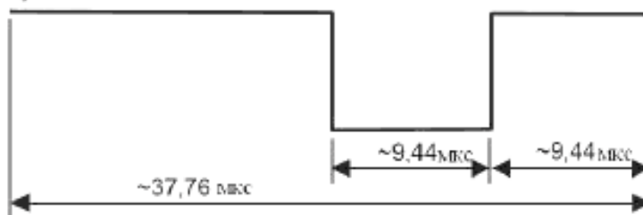
Рисунок 9 – Конец кадра при любом способе кодирования
