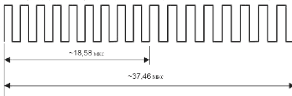
Рисунок 13 – Логическая единица при использовании двух поднесущих
