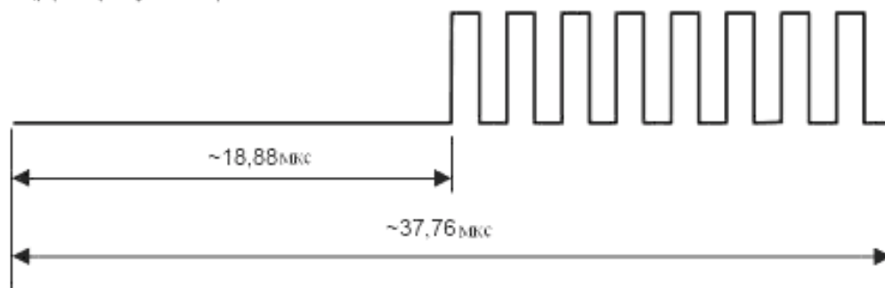
Рисунок 11 – Логическая единица
