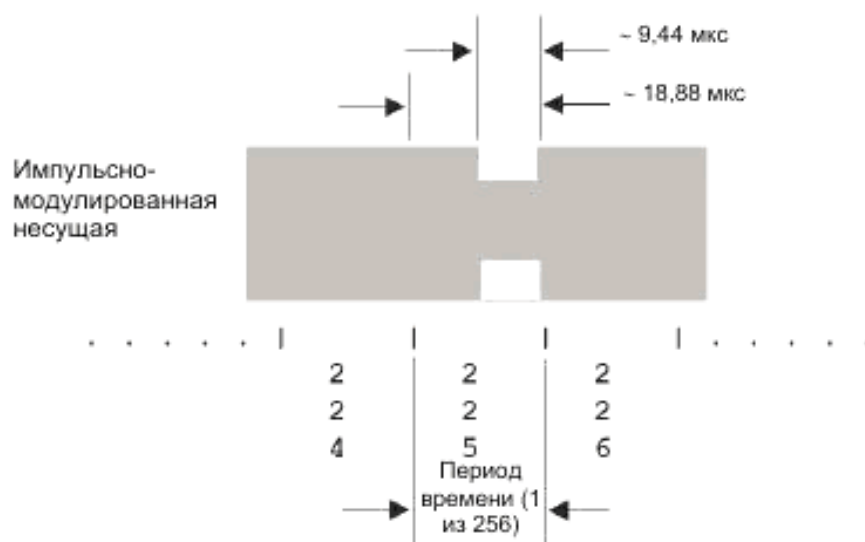
Рисунок 4 – Параметры одного периода
