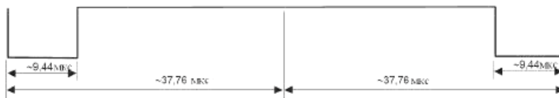
Рисунок 7 – Начало кадра при способе кодирования «1 из 256»
