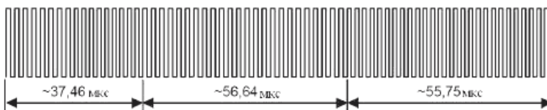
Рисунок 17 – Конец кадра при использовании двух поднесущих
