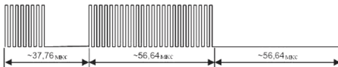
Рисунок 16 – Конец кадра при использовании одной поднесущей
