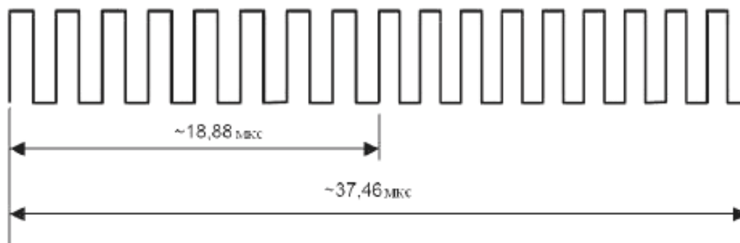
Рисунок 12 – Логический ноль при использовании двух поднесущих
