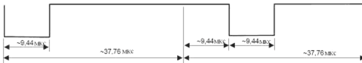
Рисунок 8 – Начало кадра при способе кодирования «1 из 4»
