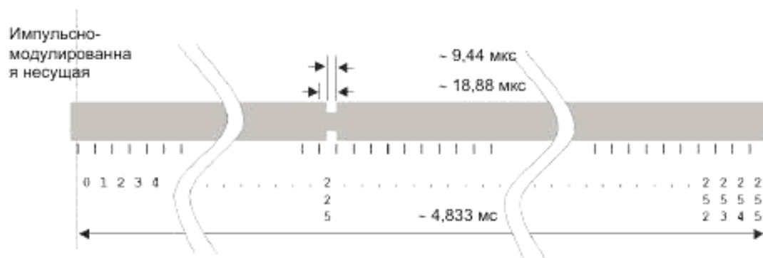
Рисунок 3 – Способ кодирования «1 из 256»
