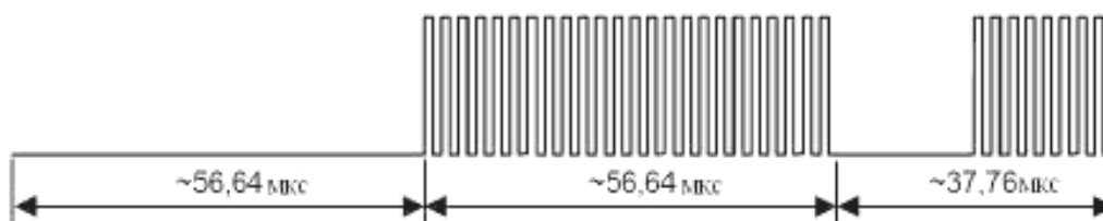
Рисунок 14 – Начало кадра при использовании одной поднесущей
