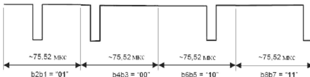
Рисунок 6 – Пример кодирования способом «1 из 4»
