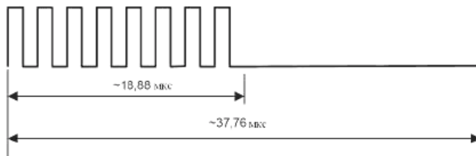
Рисунок 10 – Логический ноль
