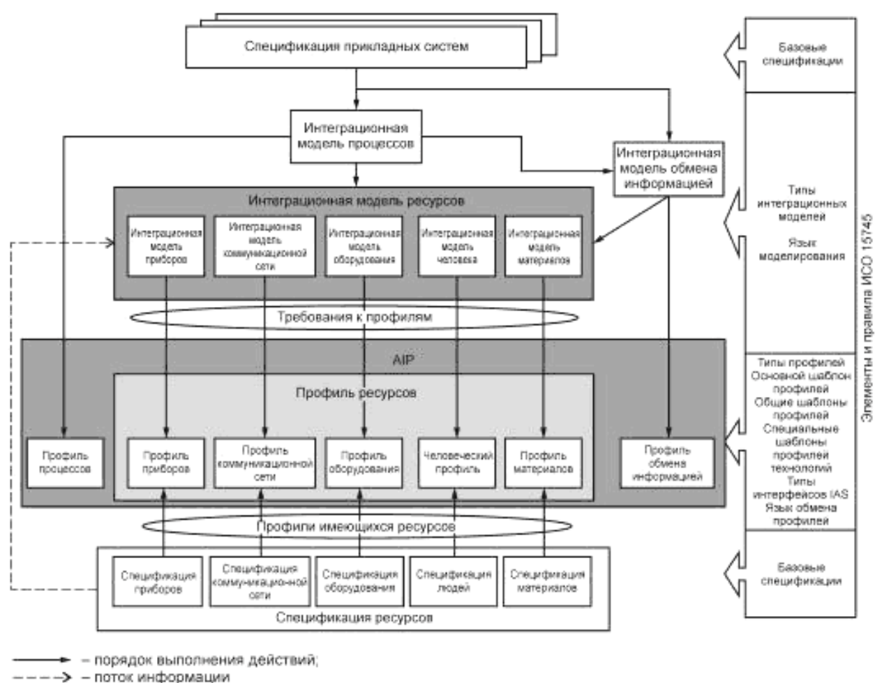
Рисунок 2 — Разработка профилей на основе ИСО 15745
