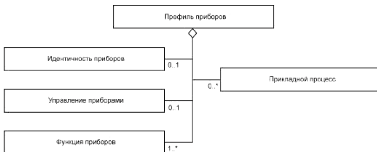
Рисунок 12 — Диаграмма класса общего профиля приборов
