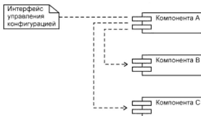
Рисунок В.1 — Пример диаграммы компонентов CMI
