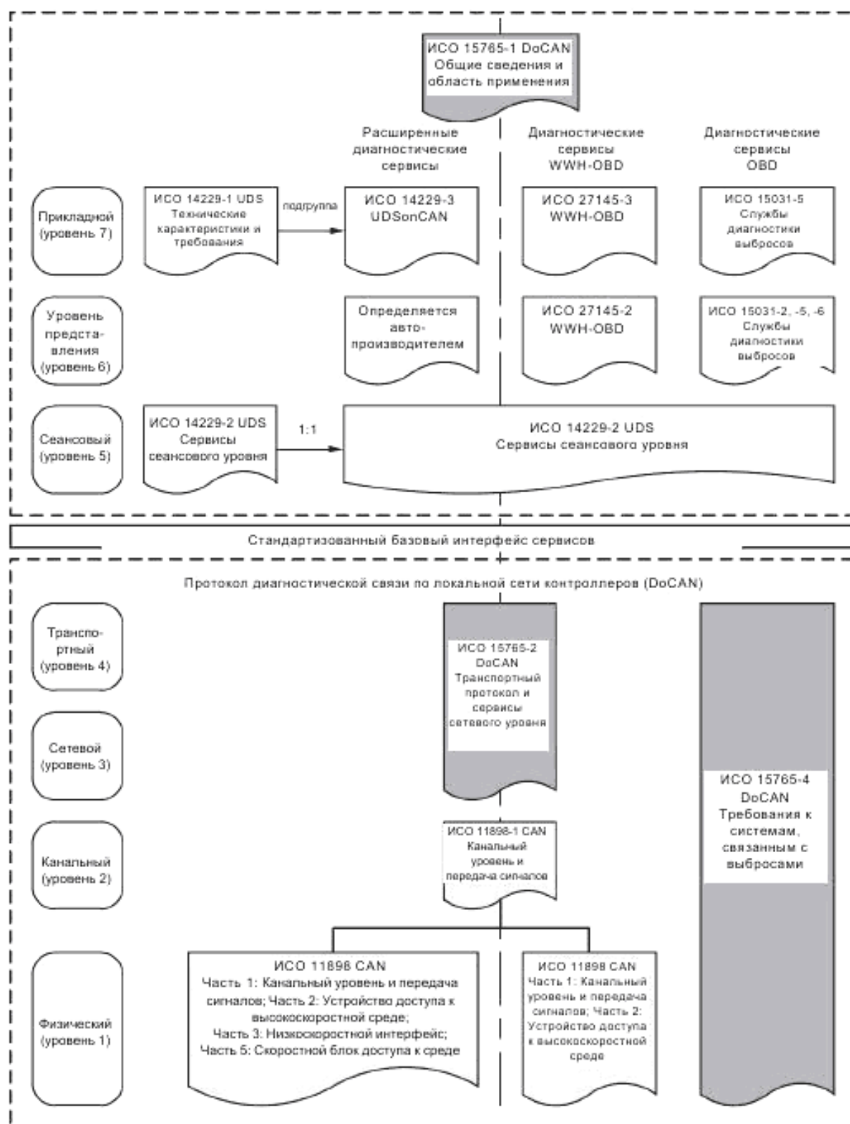
Рисунок 1 – Представление диагностической связи по локальной сети контроллеров на основании модели ВОО
