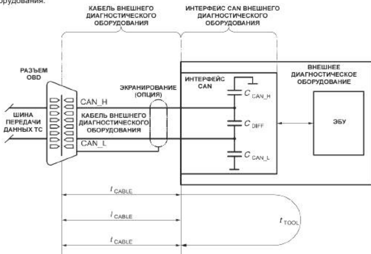
Рисунок 9 – Электротехнические параметры внешнего диагностического оборудования
