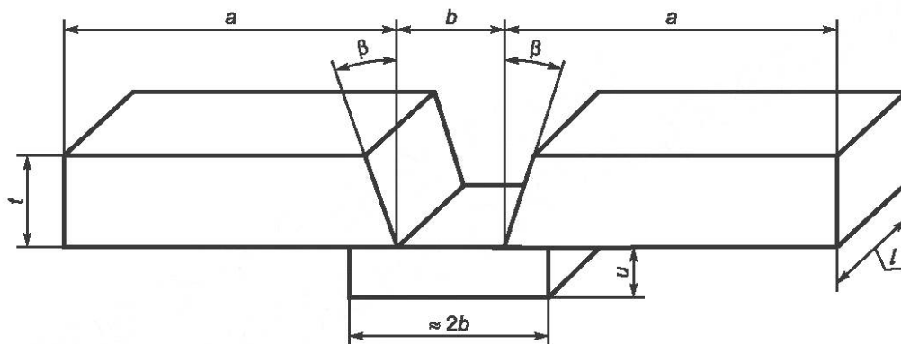
Рисунок 1 — Размеры заготовки
